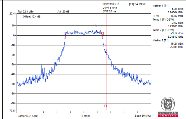
802.11ac(VHT20)_Chain1 / CH48
