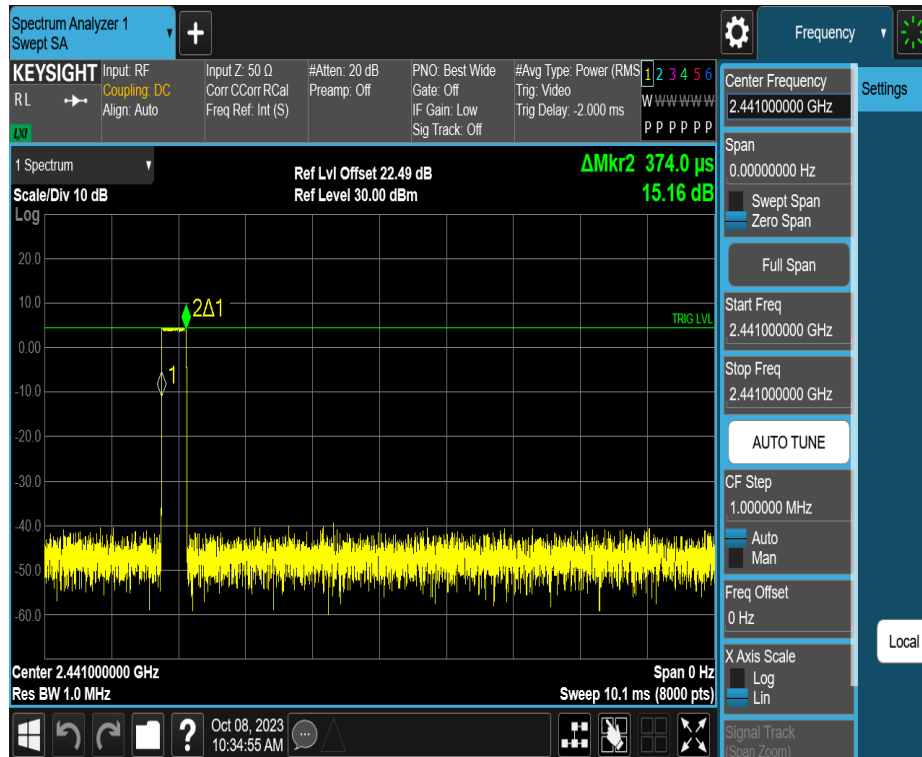
DH1_Ant1_Hop
