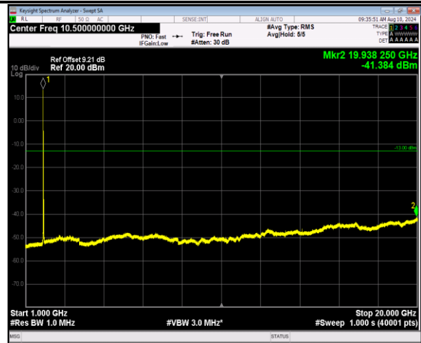
2-2-5MHz-20MHz-QPSK-QPSK-18633-18750-1RB#0-1RB# 99-1000~20000MHz-PASS
