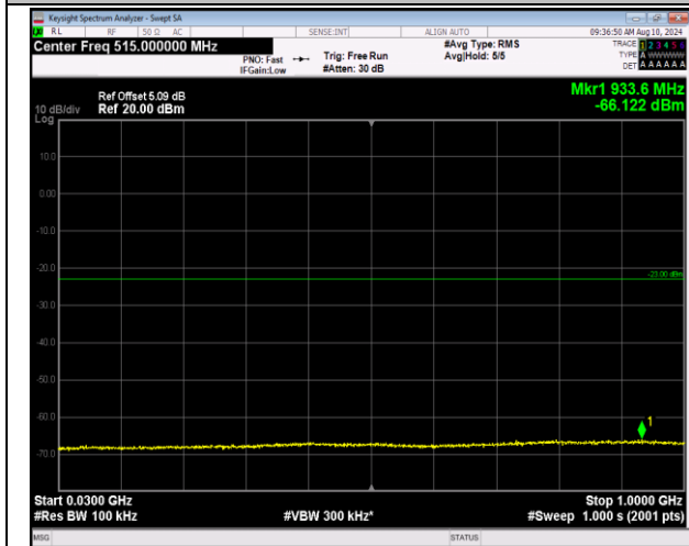
2-2-5MHz-20MHz-QPSK-QPSK-18633-18750-25RB#0-1 00RB#0-30~1000MHz-PASS
