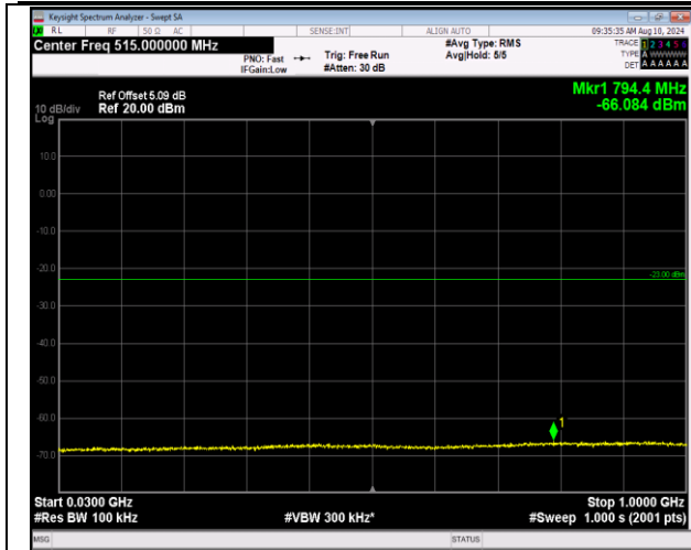
2-2-5MHz-20MHz-QPSK-QPSK-18633-18750-1RB#0-1R B#99-30~1000MHz-PASS
