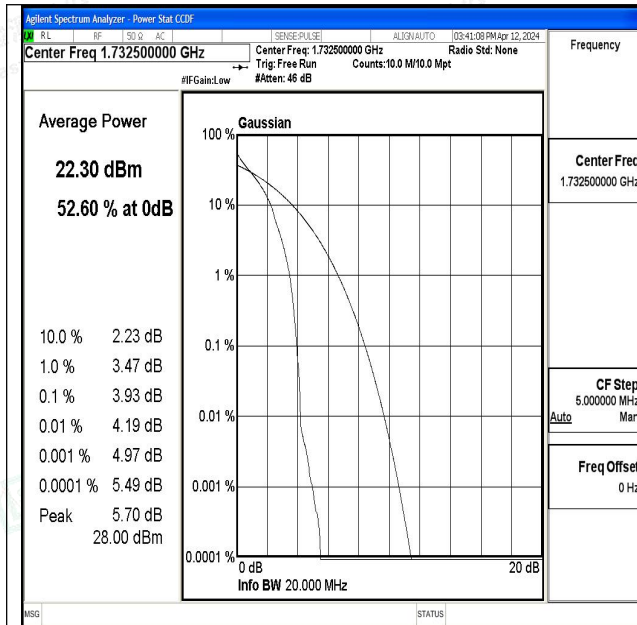
Band4-20MHz-QPSK-20175-1RB#0-PASS
