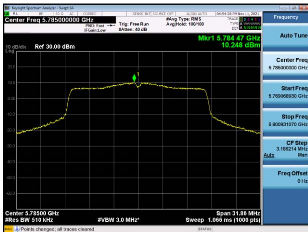
802.11ax HE20 (CH 157 : 5785 MHz) – Chain 0
