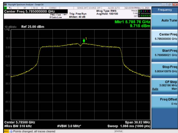
802.11ax HE20 (CH 157 : 5785 MHz) – Chain 1
