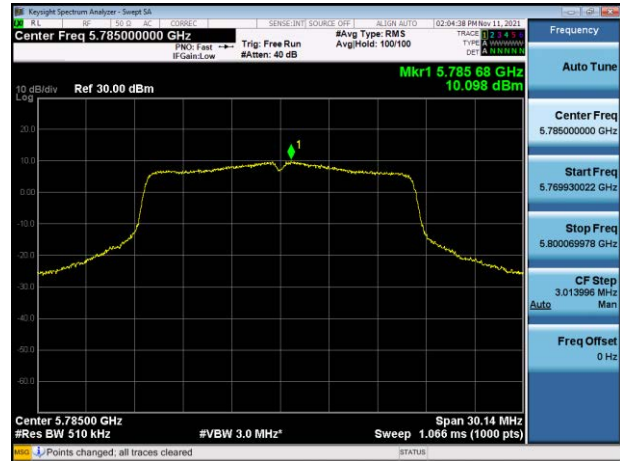
802.11n HT20 (CH 157 : 5785 MHz) – Chain 1
