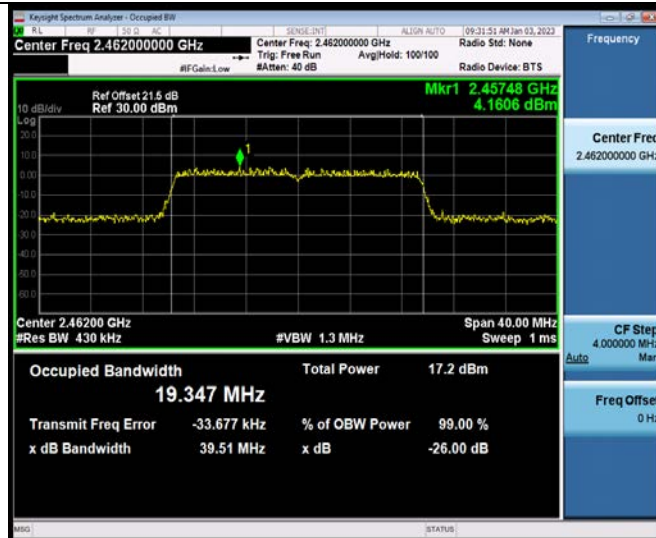
11AX20MIMO_Ant2_2462
