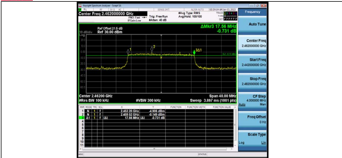
11N20MIMO_Ant2_2462
