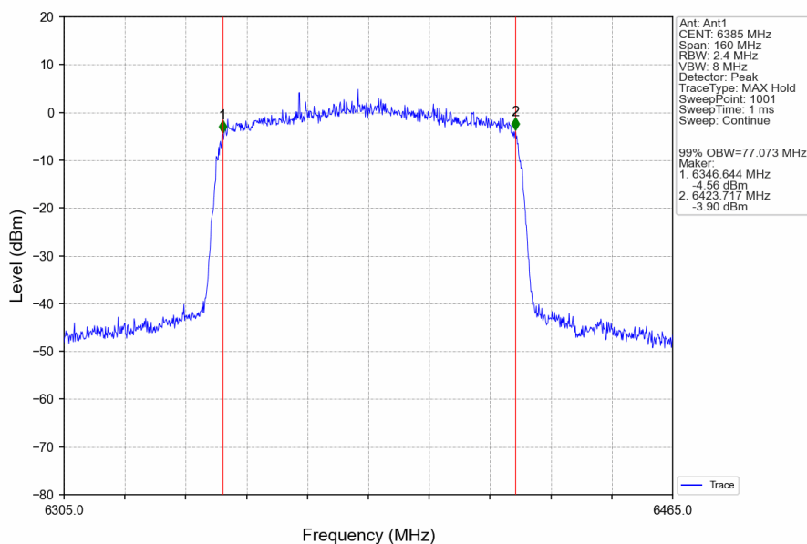
802.11ax(HEW80)_HCH_6385MHz_RU996_Left_Ant1_NTNV
