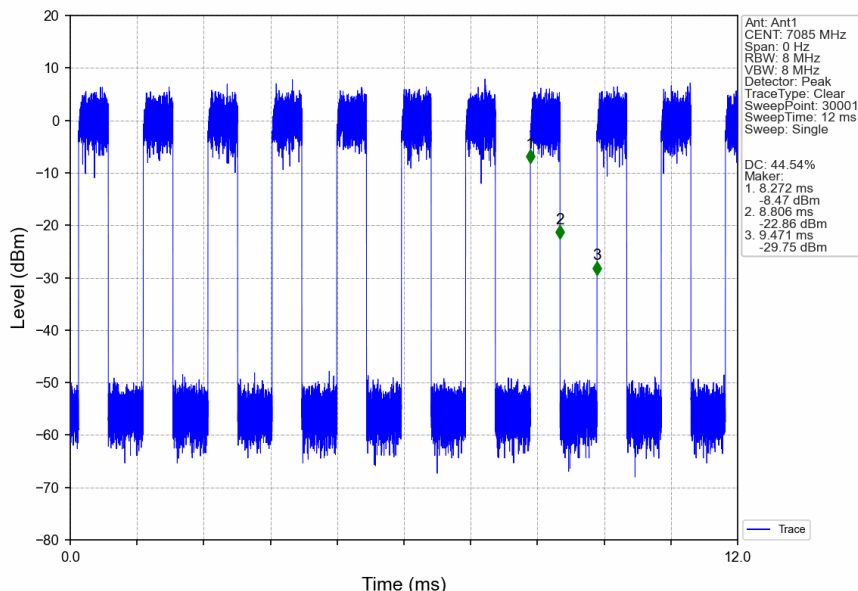
802.11ax(HEW40)_HCH_7085MHz_RU484_Left_Ant1_NTNV
