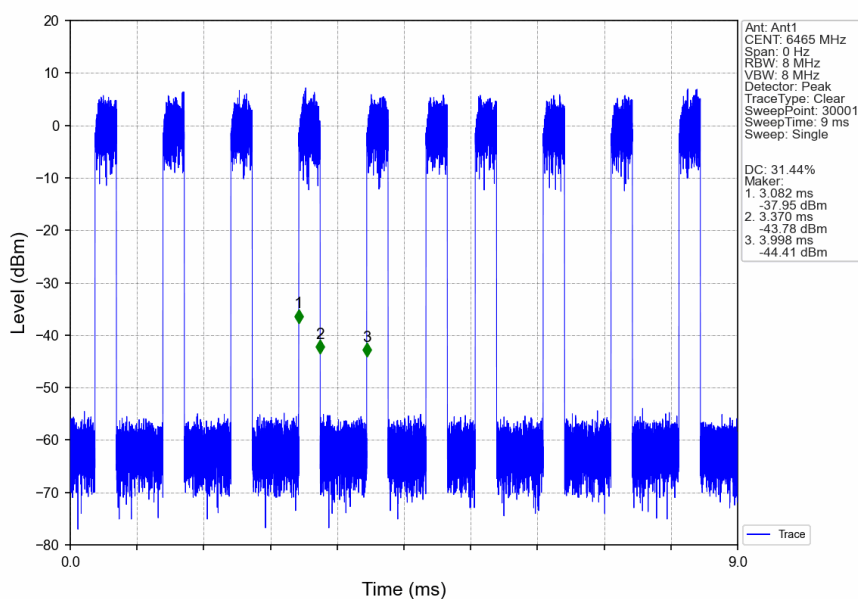
802.11ax(HEW80)_LCH_6465MHz_RU996_Left_Ant1_NTNV
