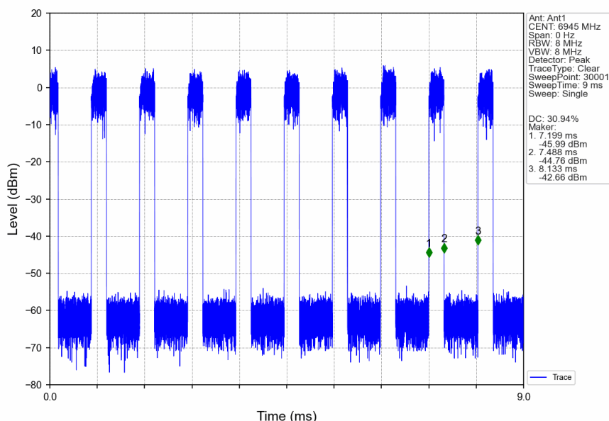
802.11ax(HEW80)_LCH_6945MHz_RU996_Left_Ant1_NTNV
