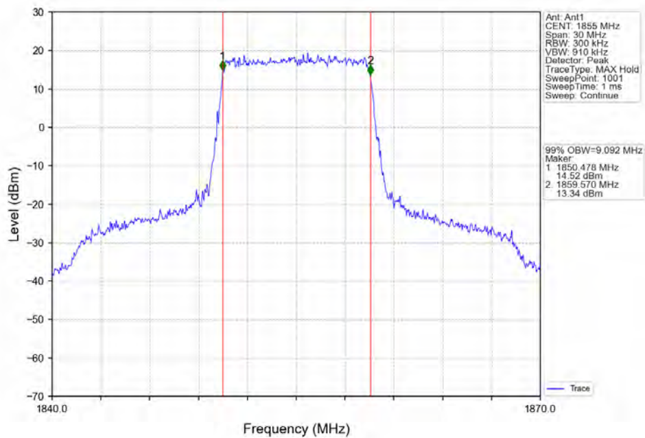
Band25_10MHz_QPSK_LCH_1855MHz_RB_50_0 NTN
