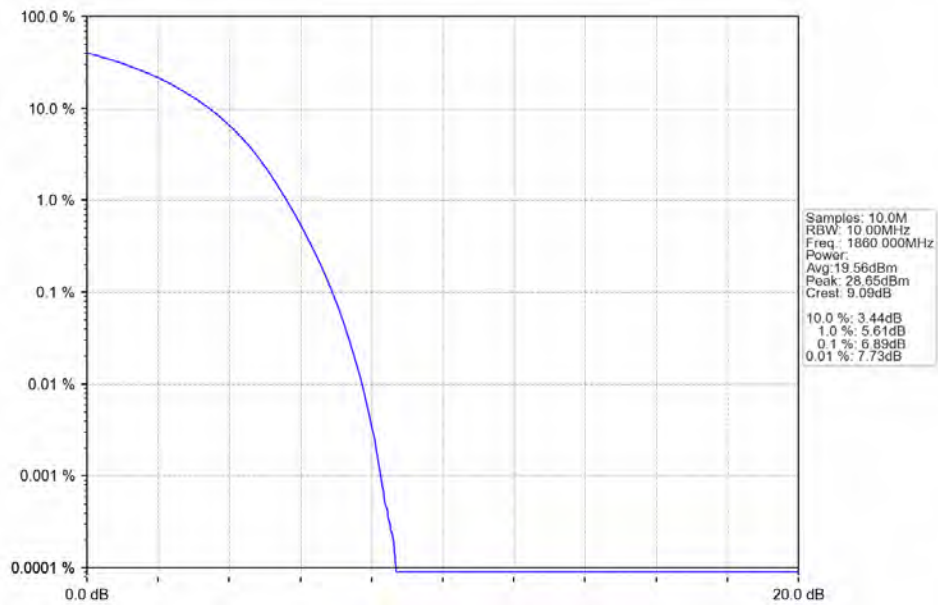
Band25 20MHz 64QAM LCH 1860MHz RB 100 0 NTN
