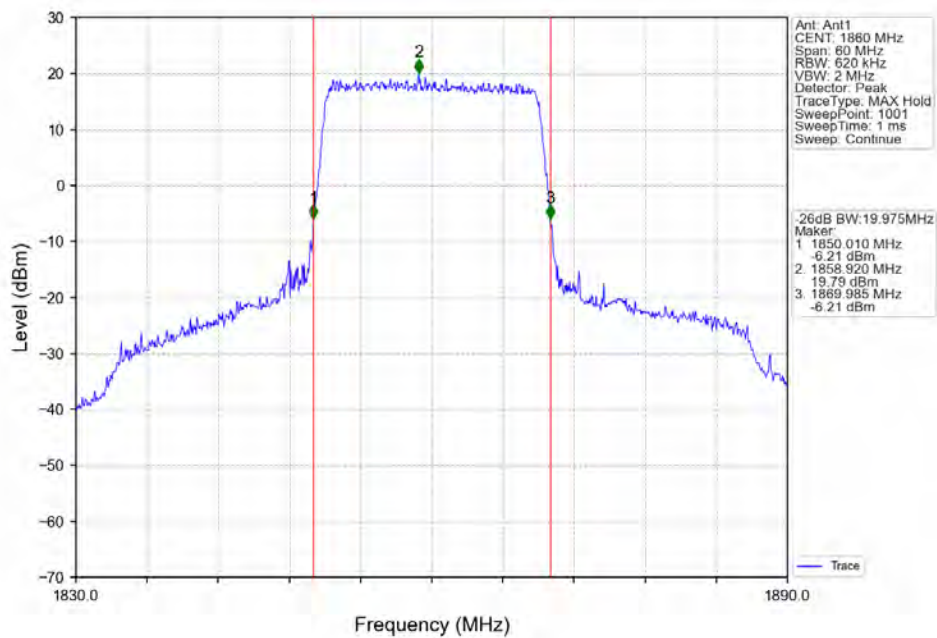
Band25_20MHz_QPSK_LCH_1860MHz_RB_100_0_NTNV
