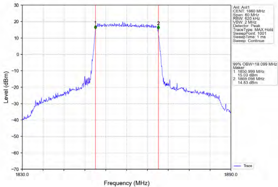
Band25_20MHz_QPSK_LCH_1860MHz_RB_100_0_NTNV
