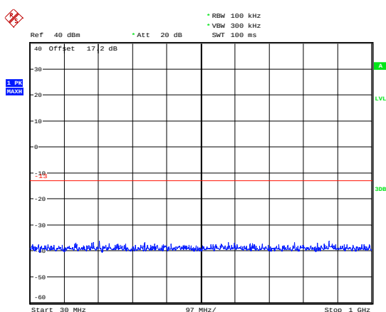
GSM 1900 CH- Middle 30MHz ~ 1GHz
