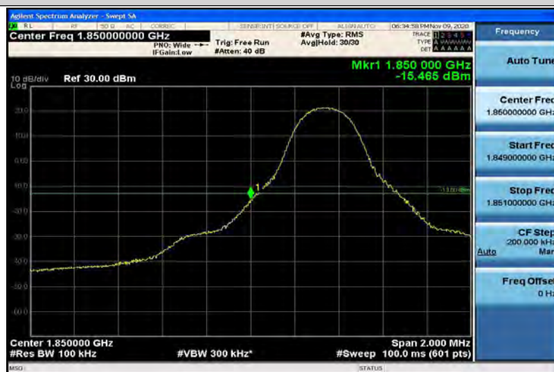
Band2-5MHz-QPSK-18625-1RB#24
