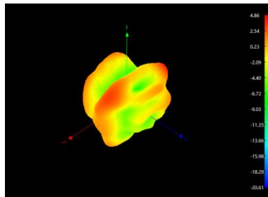
2500MHz
