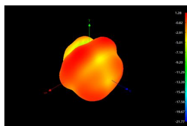
2450MHz
