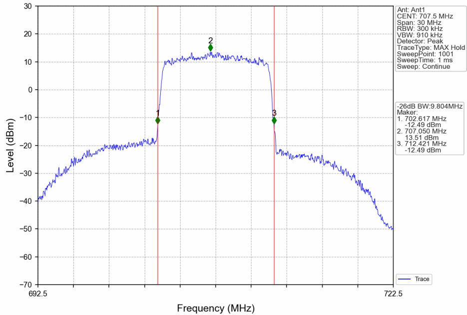
Band12_10MHz_QPSK_MCH_707.5MHz_RB_50_0_NTNV
