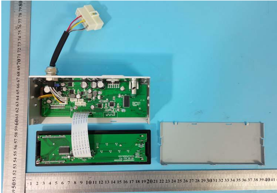
(2) EUT Photo
