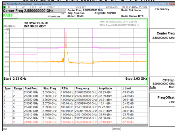
Band38_20MHz_CP_OFDM_SCS30kHz_QPSK_RB1_50_CH516000
