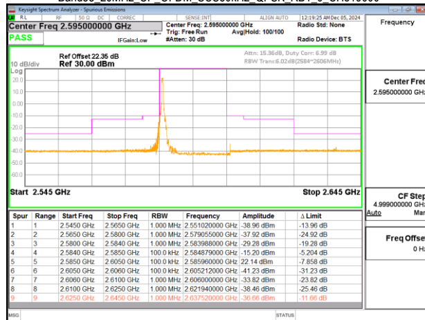
Band38_20MHz_CP_OFDM_SCS30kHz_QPSK_RB1_50_CH519000
