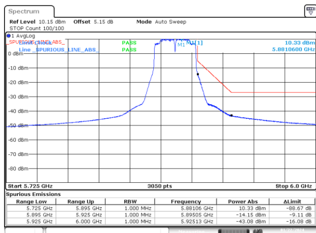
BE-NR-HIGH, MIMO-B, 802.11n40-HT0, Ch175
