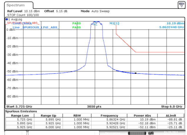
BE-NR-HIGH, MIMO-A, 802.11n20-HT0, Ch173
