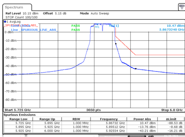
BE-NR-HIGH, MIMO-A, 802.11n40-HT0, Ch175
