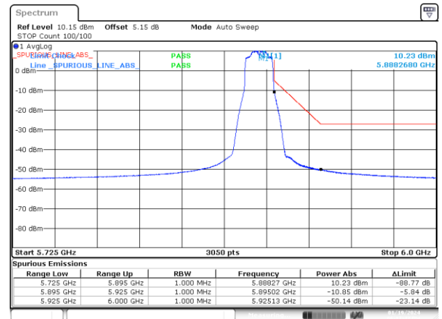
BE-NR-HIGH, MIMO-A, 802.11n20-HT0, Ch177
