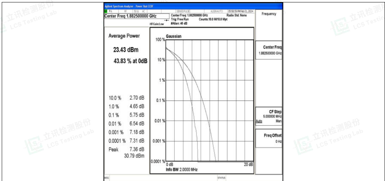
Band25-1.4MHz-QPSK-26365-6RB#0-PASS
