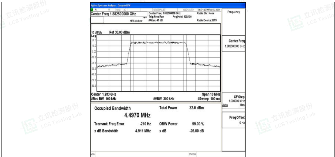
Band25-5MHz-QPSK-26365-25RB#0-PASS
