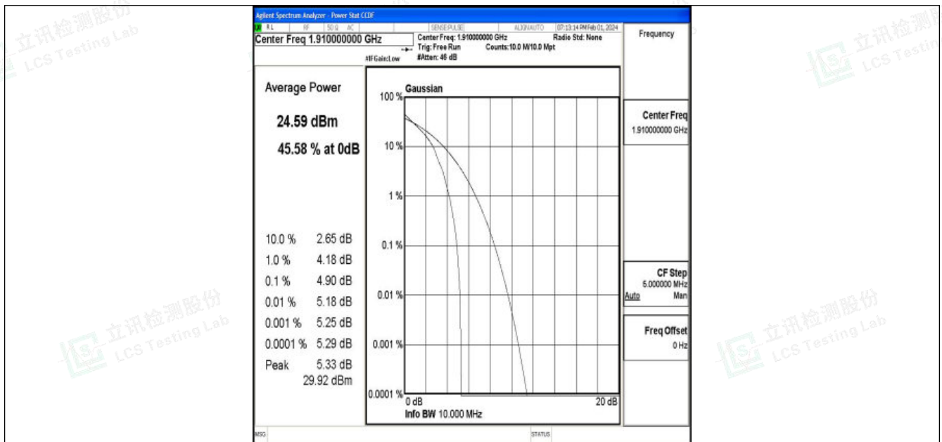
Band25-10MHz-QPSK-26640-1RB#0-PASS
