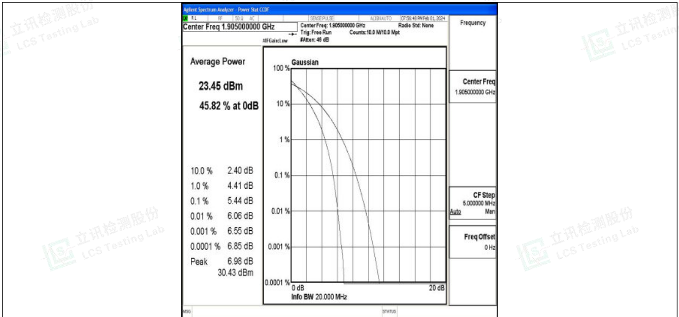
Band25-20MHz-QPSK-26590-100RB#0-PASS
