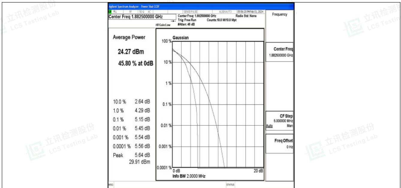
Band25-1.4MHz-QPSK-26365-1RB#0-PASS
