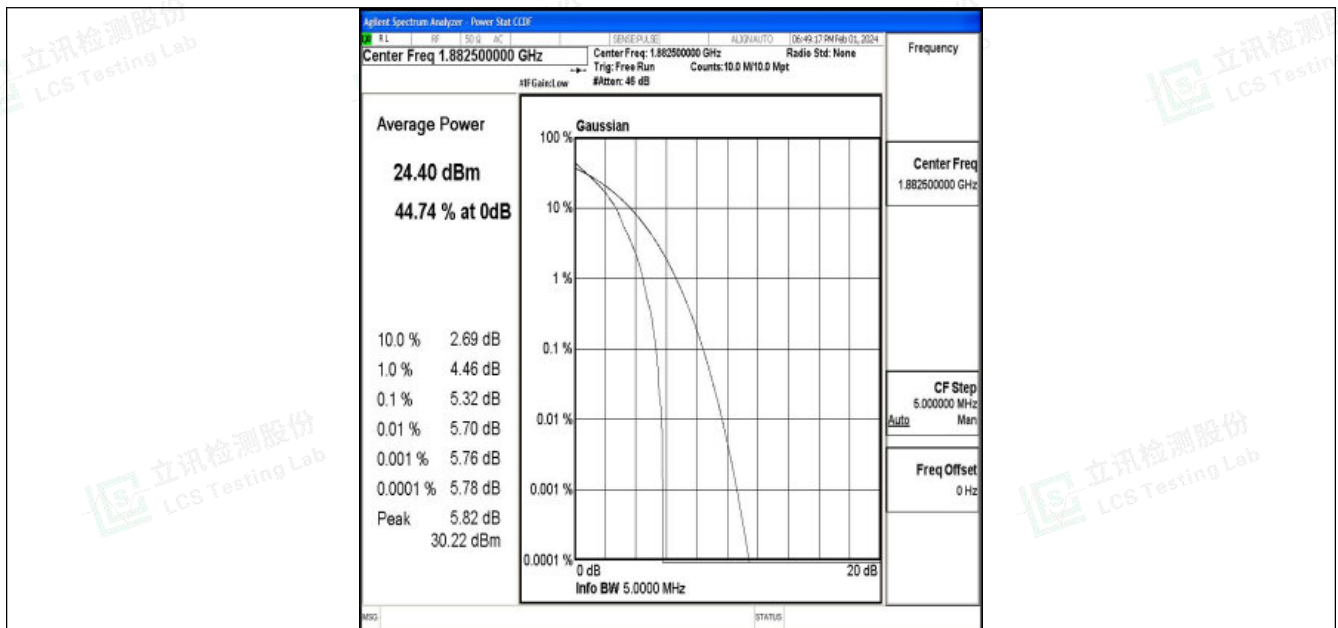
Band25-5MHz-QPSK-26365-1RB#0-PASS
