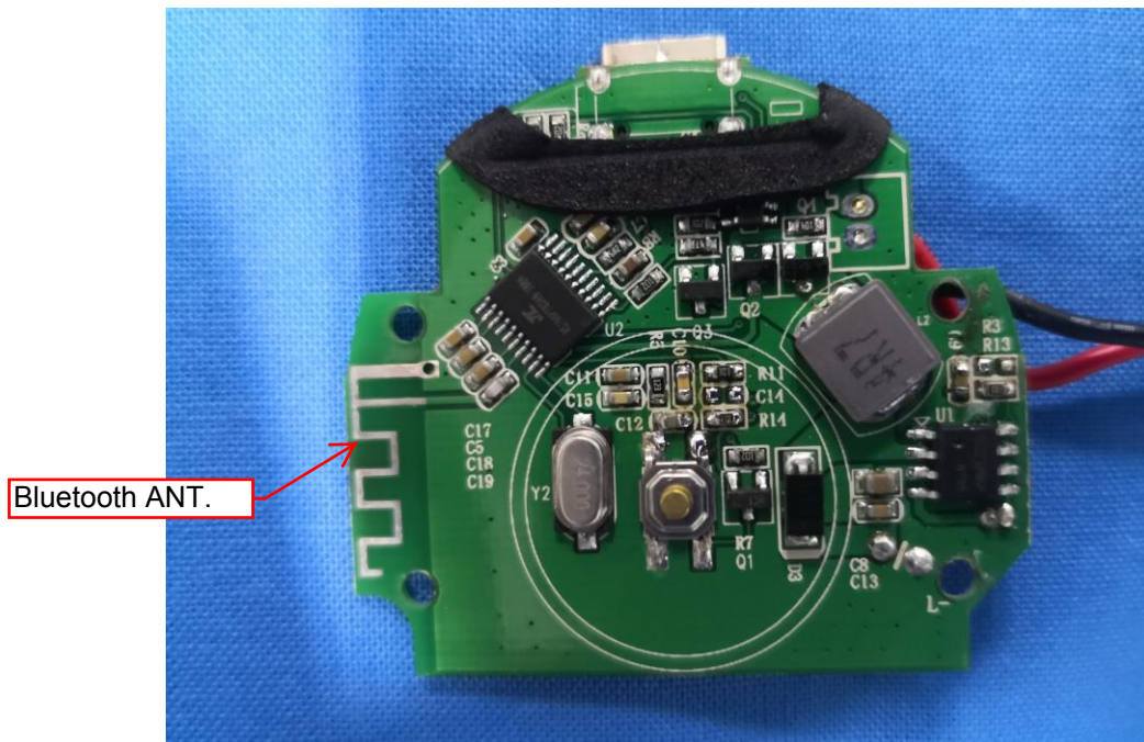
EUT Photo (10)
