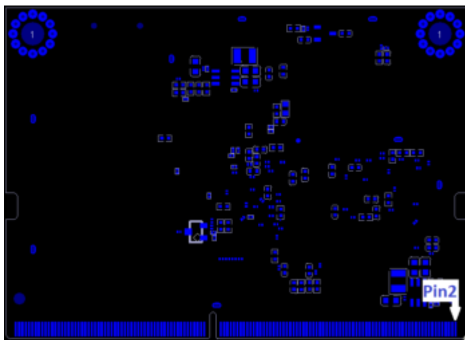
< BOT VIEW >
