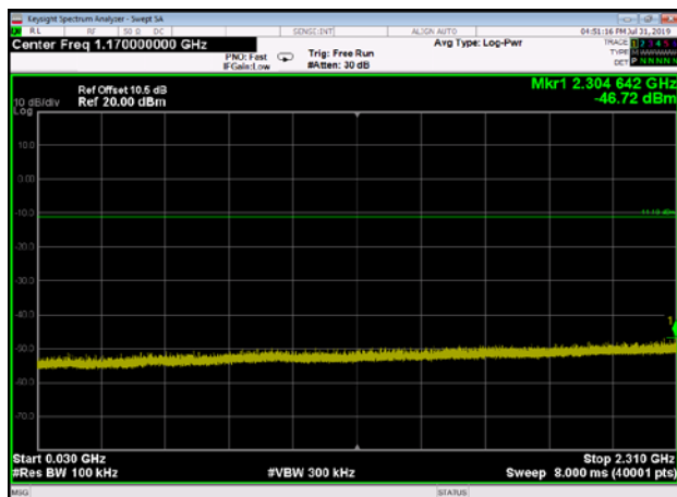
,Plot 3,30MHz~2310MHz-802.11b,2462MHz
