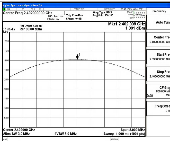
DH5_Ant1_2402
