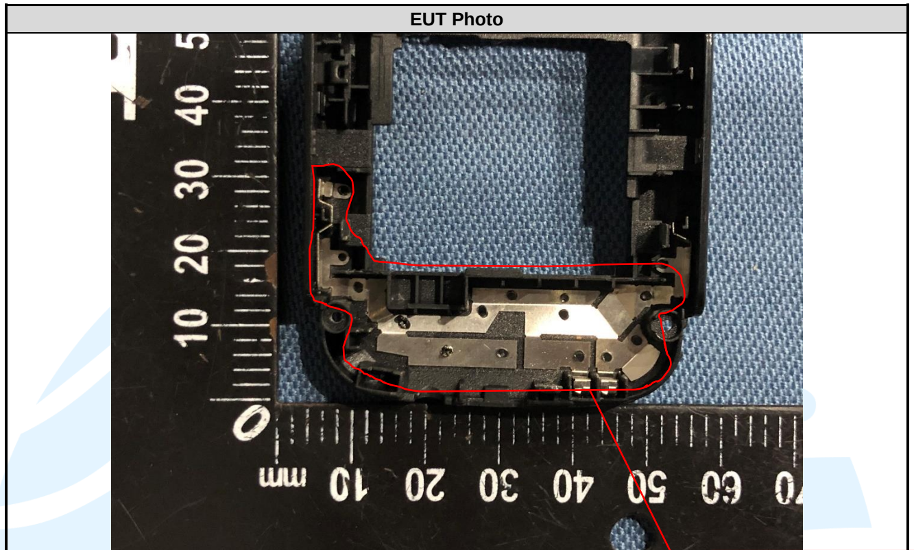
GSM Antenna
