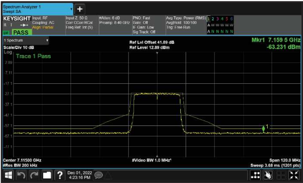
Figure 79 - B (Core 1) 802.11ax HE20 SU 7115 MHz (CH233)
