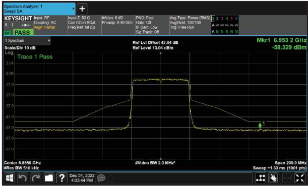
Figure 80 - B (Core 1) 802.11ax HE40 SU 6885 MHz (CH187)
