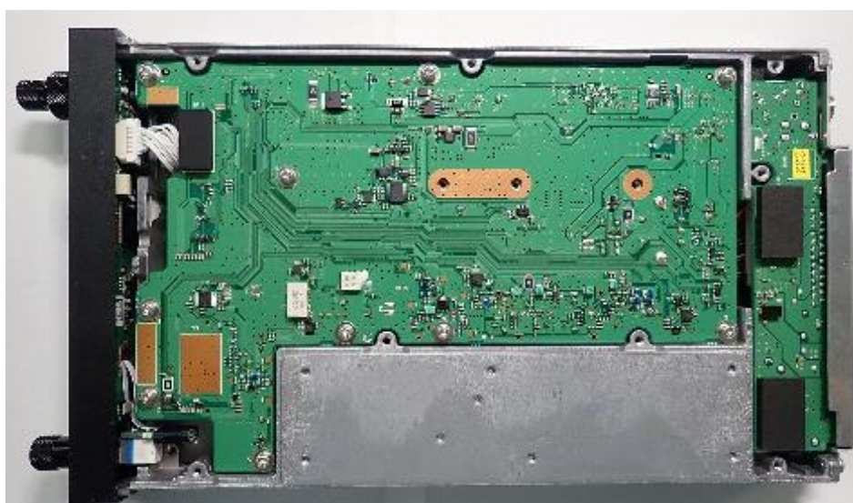
BOTTOM
