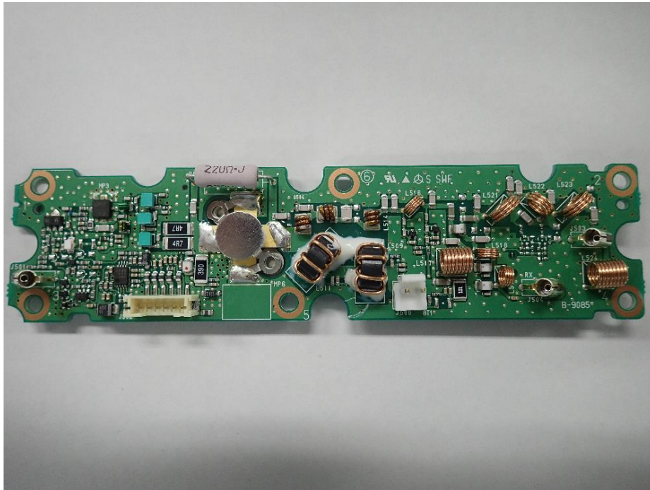
PA-D(TOP)
