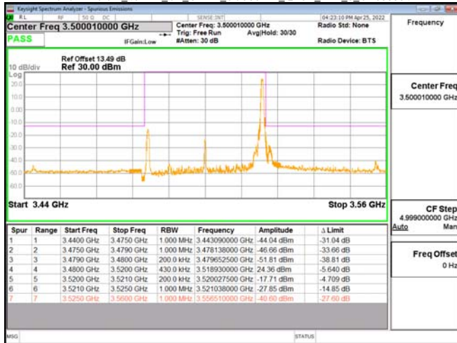
Band77-Part27_40MHz_CP_OFDM_SCS30kHz_QPSK_RB1_0_CH635332
