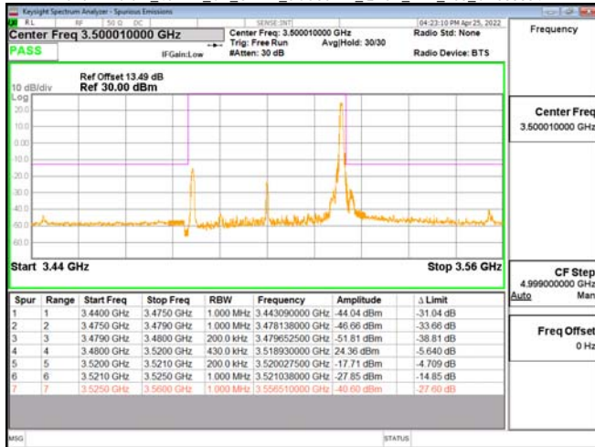
Band77-Part27_40MHz_CP_OFDM_SCS30kHz_OPSK_RB1_105_CH633332
