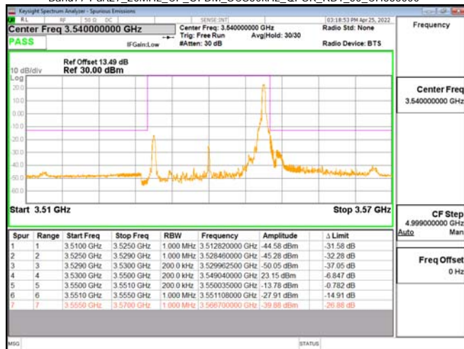
Band77-Part27_20MHz_CP_OFDM_SCS30kHz_QPSK_RB1_50_CH636000
