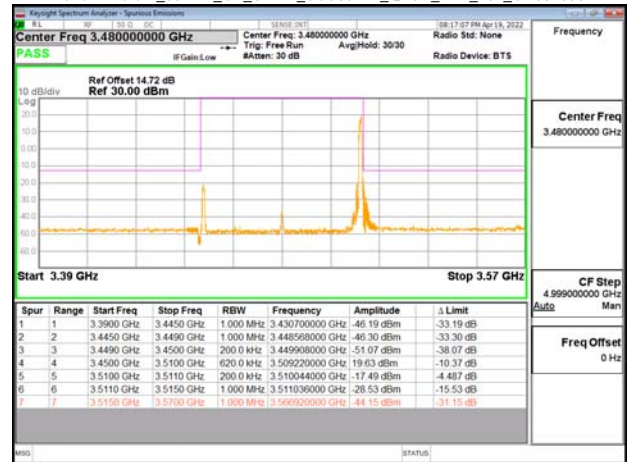
Band77-Part27_60MHz_CP_OFDM_SCS30kHz_QPSK_RB1_161_CH633334
