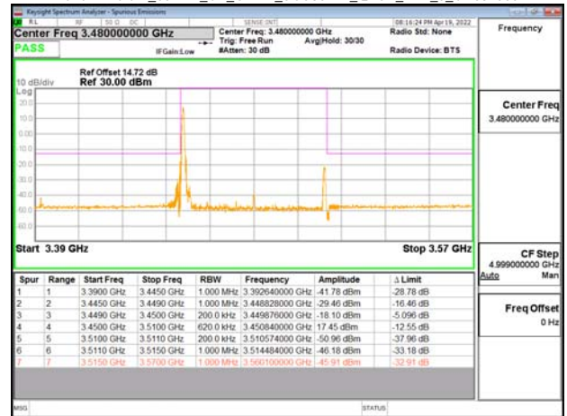
Band77-Part27_60MHz_CP_OFDM_SCS30kHz_OPSK_RB1_0_CH633334
