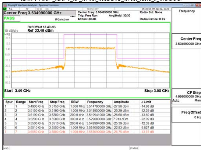
Band77-Part27_30MHz_CP_OFDM_SCS30kHz_QPSK_RB78_0_CH635666
