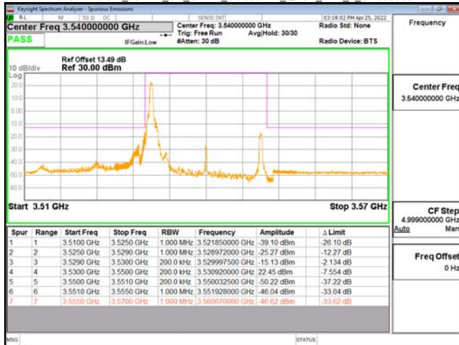
MIMO Band77-Part27_20MHz_CP_OFDM_SCS30kHz_QPSK_RB1_0_CH636000
