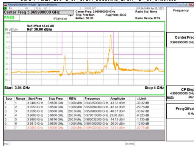
Band77-Part27_20MHz_CP_OFDM_SCS30kHz_QPSK_RB1_50_CH664666
