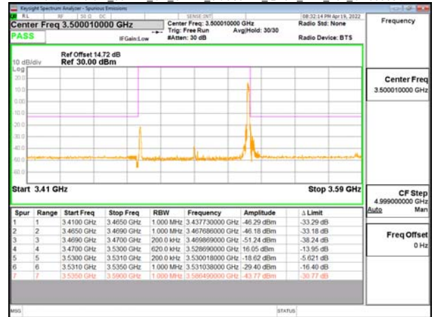
Band77-Part27_60MHz_CP_OFDM_SCS30kHz_QPSK_RB1_161_CH633334
