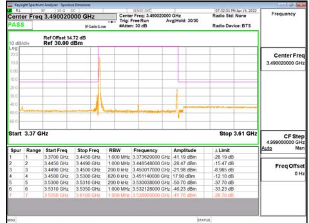
Band77-Part27_80MHz_CP_OFDM_SCS30kHz_QPSK_RB1_0_CH633334
