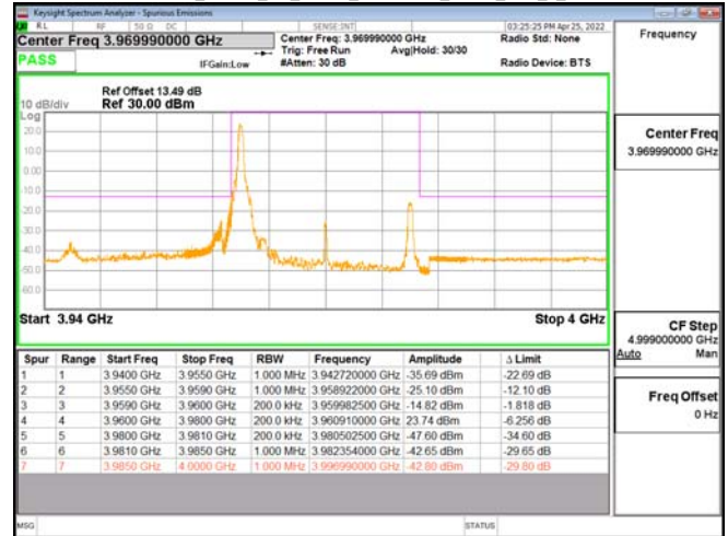
MIMO Band77-Part27_20MHz_CP_OFDM_SCS30kHz_QPSK_RB1_0_CH64666
