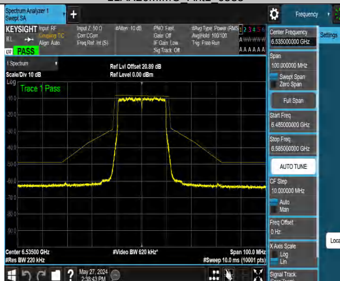
11AX20MIMO_Ant1_6535
