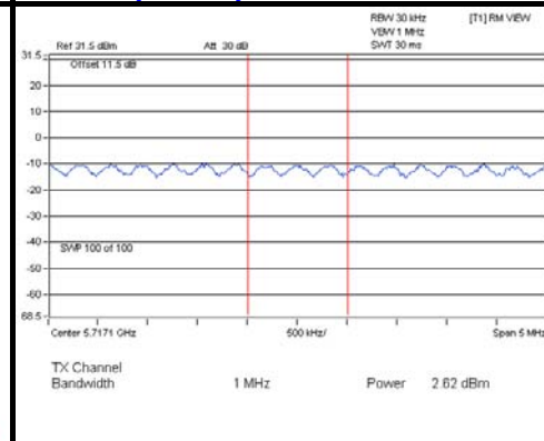
802.11ac (80MHz)
