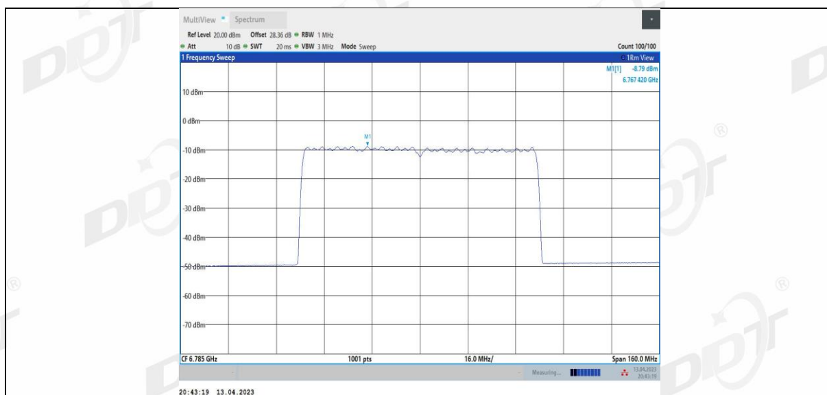
11AX80MIMO_Ant4_6785
