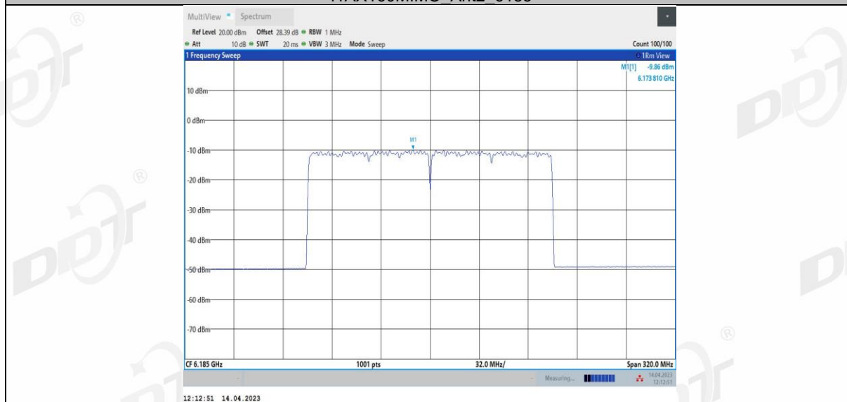
11AX160MIMO Ant3 6185
