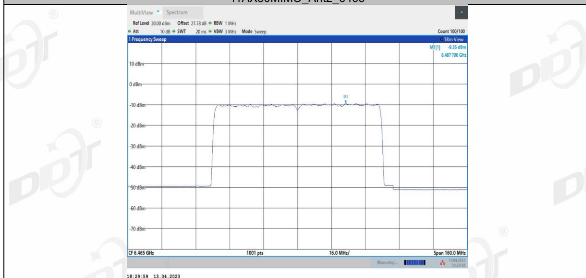
11AX80MIMO_Ant3_6465
