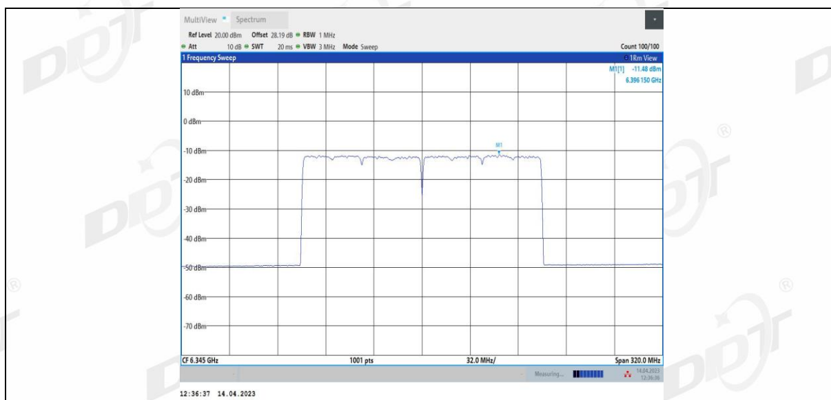
11AX160MIMO Ant4 6345
