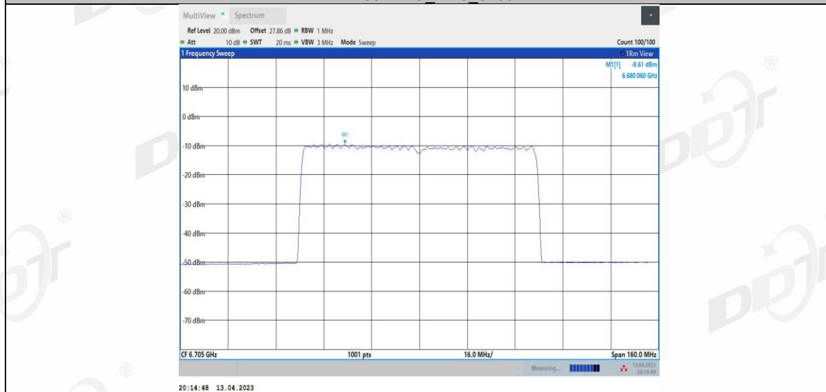
11AX80MIMO_Ant4_6705
