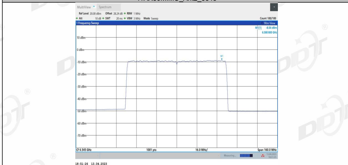
11AX80MIMO_Ant3_6545
