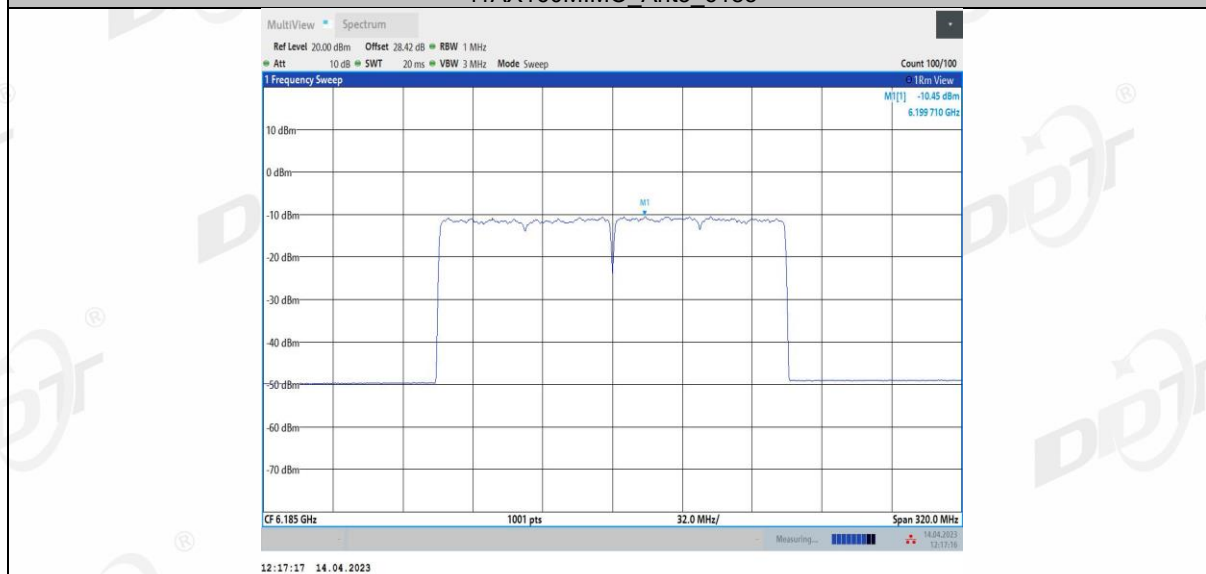
11AX160MIMO Ant4 6185
