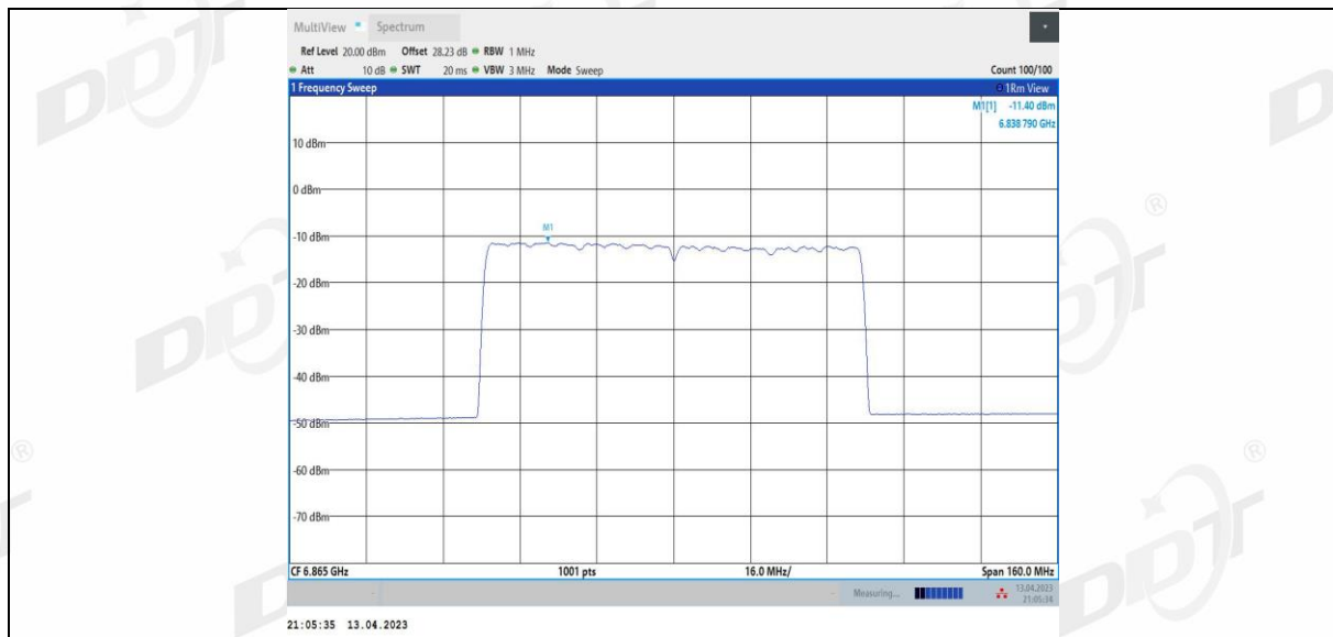
11AX80MIMO_Ant3_6865
