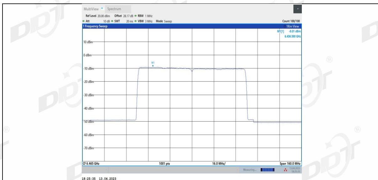
11AX80MIMO_Ant2_6465
