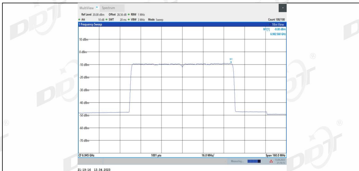
11AX80MIMO_Ant2_6945
