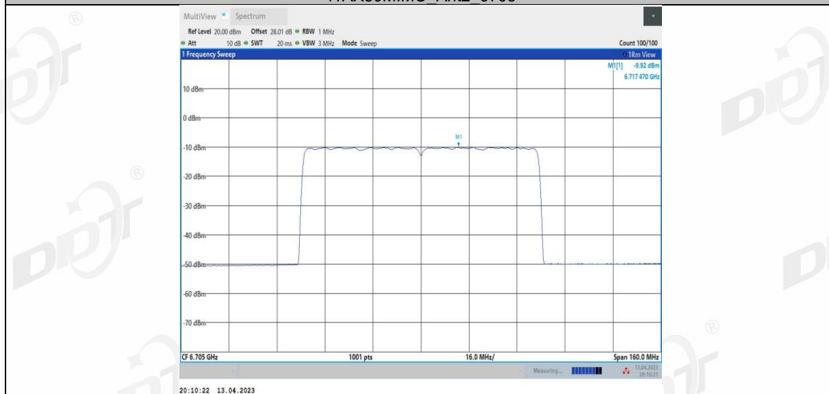
11AX80MIMO_Ant3_6705
