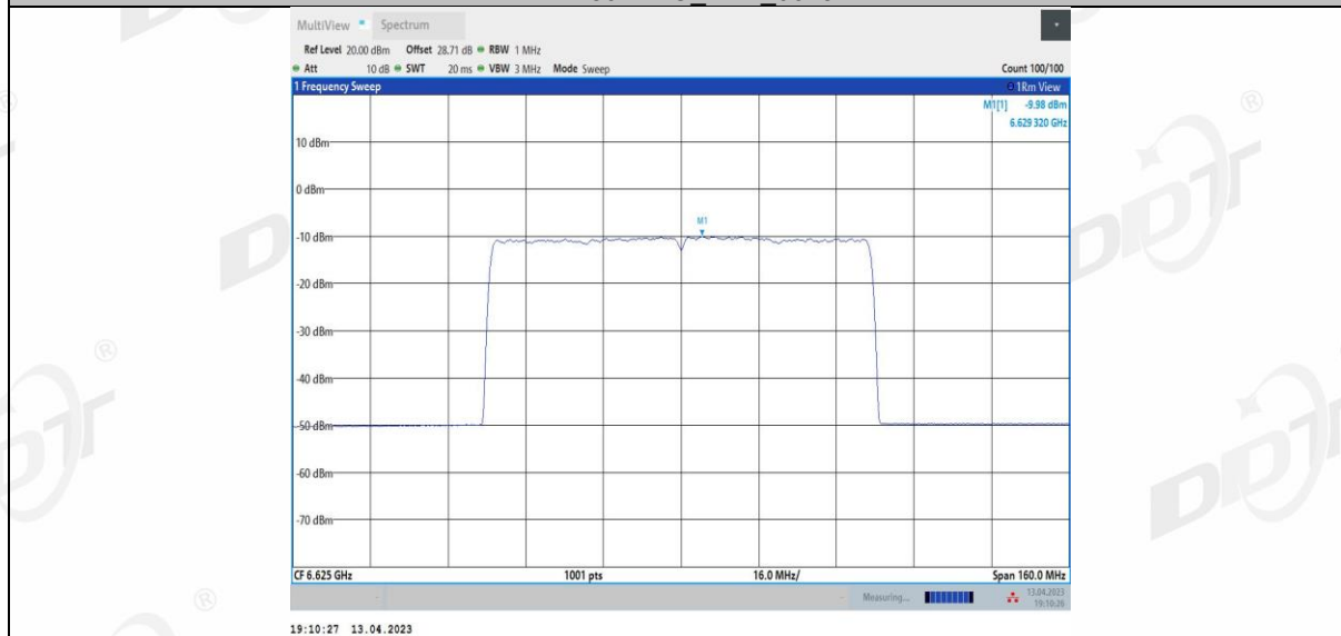
11AX80MIMO_Ant2_6625
