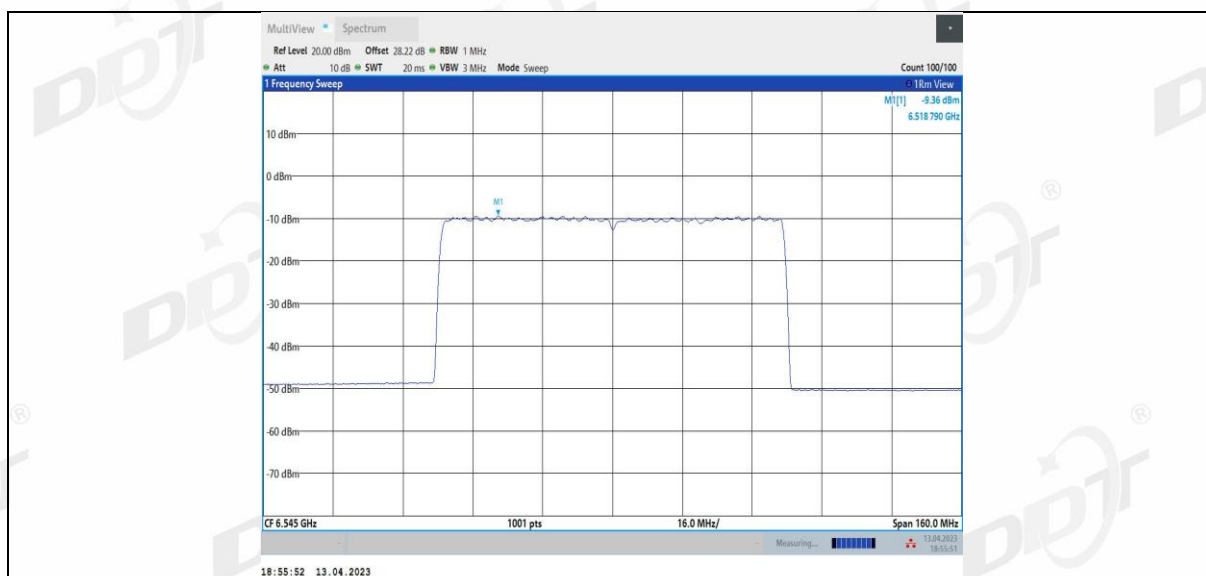
11AX80MIMO_Ant4_6545
