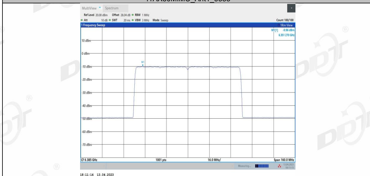
11AX80MIMO_Ant2_6385
