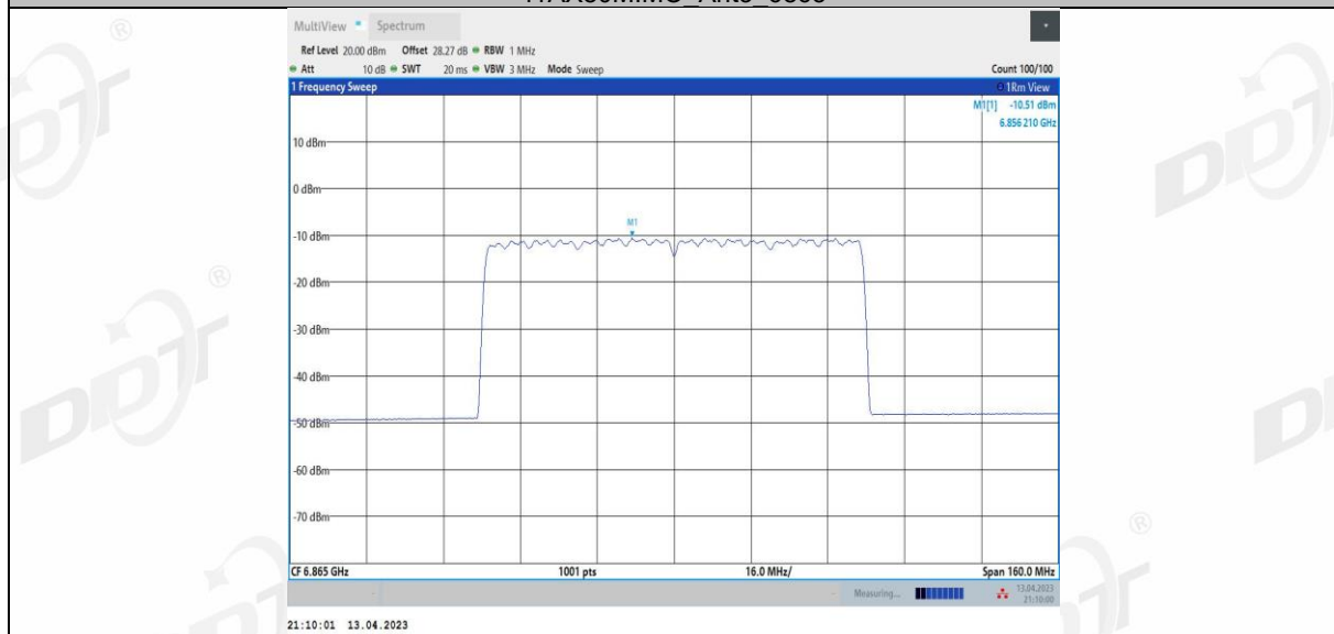
11AX80MIMO_Ant4_6865
