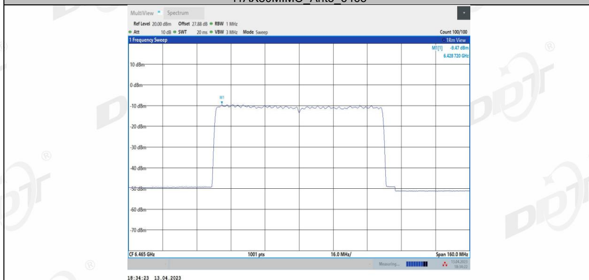
11AX80MIMO_Ant4_6465
