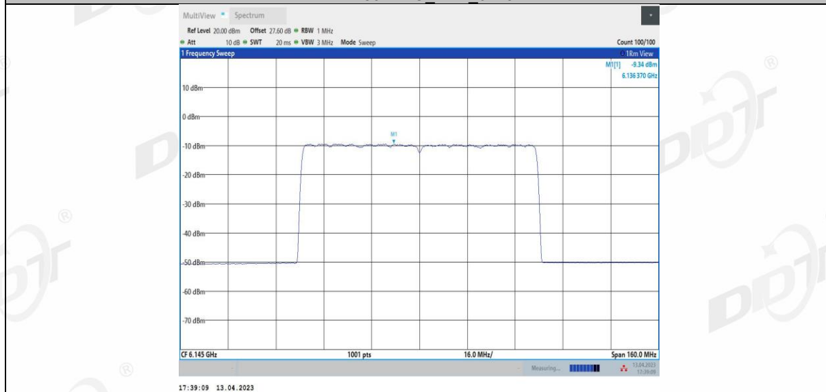
11AX80MIMO_Ant3_6145
