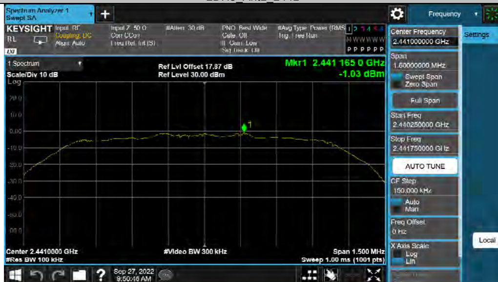
2DH5 Ant1 2441
