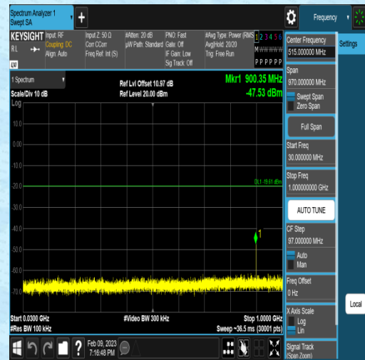
11G-Ant1-2437-30~1000-0.39
