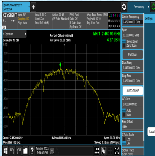
11B-Ant2-2462-Reference-4.27
