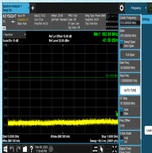
11G-Ant1-2462-30~1000-3.09
