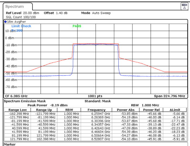
802.11ax (80MHz) 6385MHz Chain D NSS-1
