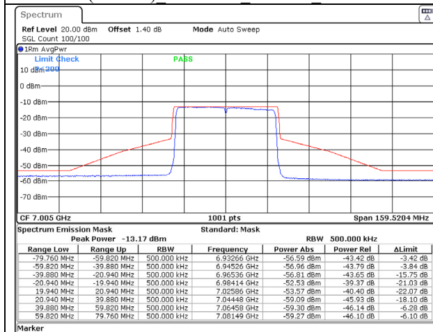
802.11ax (40MHz) 7005MHz Chain C NSS-1
