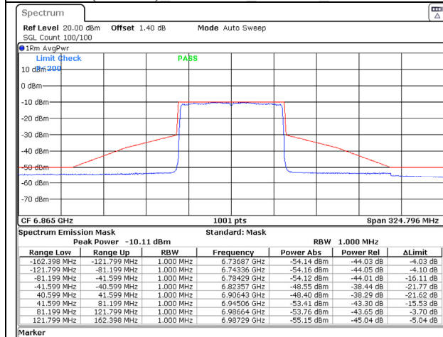
802.11ax (80MHz) 6865MHz Chain A NSS-1
