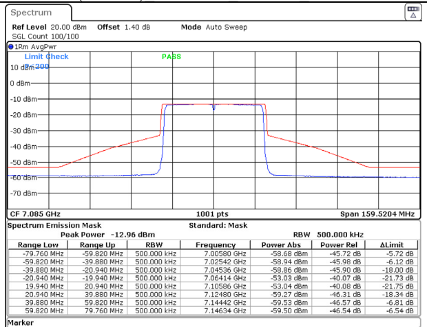
802.11ax (40MHz) 7085MHz Chain B NSS-1
