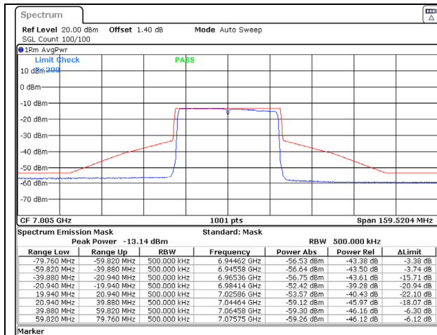
802.11ax (40MHz) 7005MHz Chain A NSS-1
