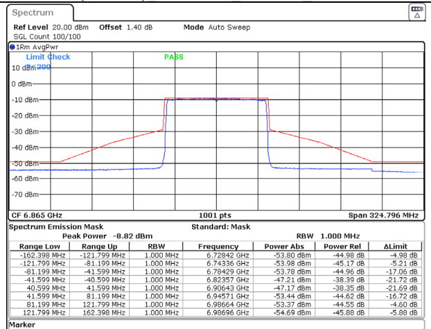
802.11ax (80MHz) 6865MHz Chain B NSS-1
