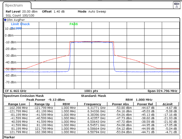
802.11ax (80MHz) 6465MHz Chain D NSS-1
