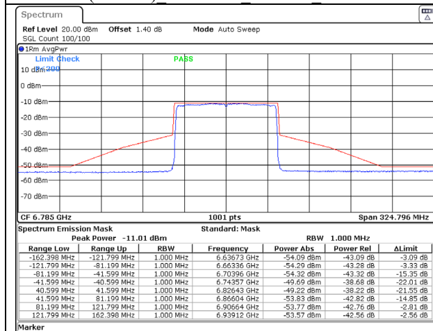
802.11ax (80MHz) 6785MHz Chain C NSS-1
