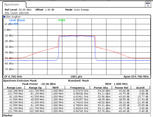
802.11ax (80MHz) 6705MHz Chain D NSS-1
