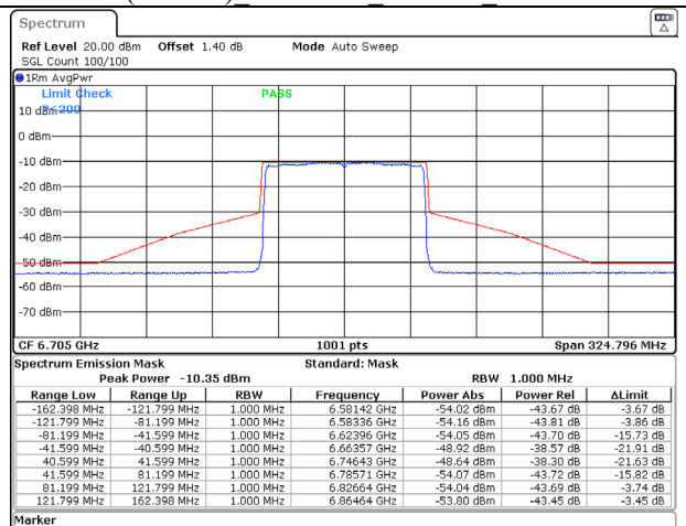
802.11ax (80MHz) 6705MHz Chain B NSS-1
