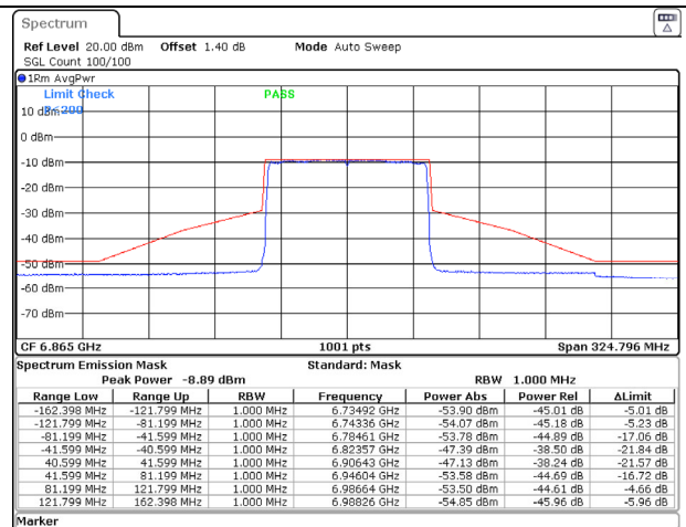
802.11ax (80MHz) 6865MHz Chain D NSS-1
