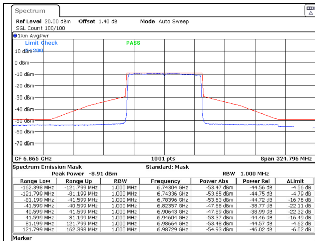
802.11ax (80MHz) 6865MHz Chain C NSS-1
