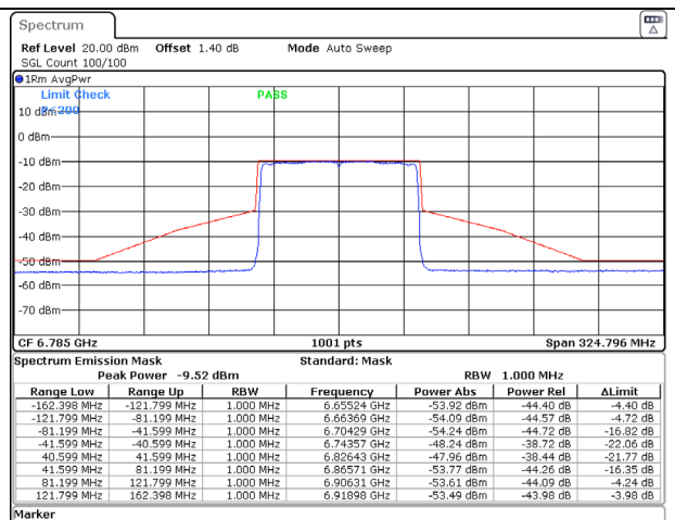
802.11ax (80MHz) 6785MHz Chain B NSS-1
