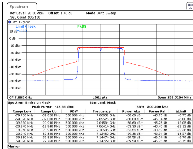
802.11ax (40MHz) 7085MHz Chain C NSS-1
