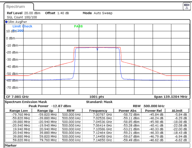
802.11ax (40MHz) 7085MHz Chain D NSS-1
