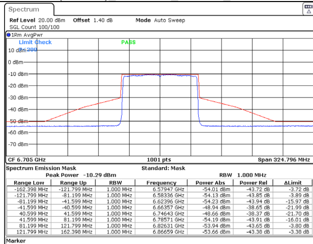
802.11ax (80MHz) 6705MHz Chain C NSS-1
