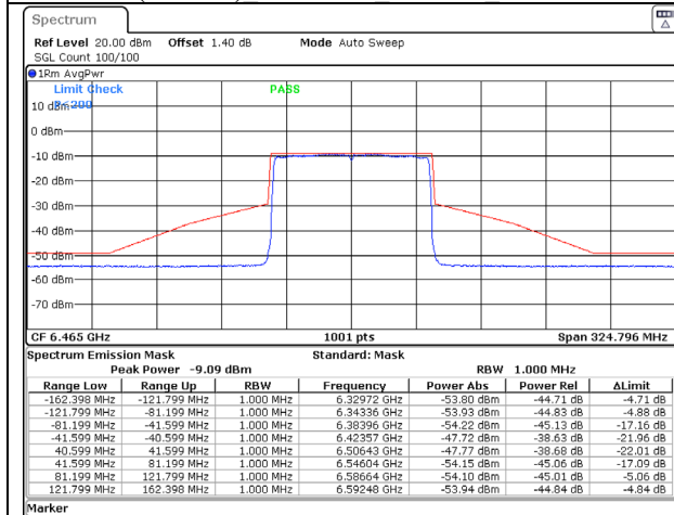
802.11ax (80MHz) 6465MHz Chain C NSS-1
