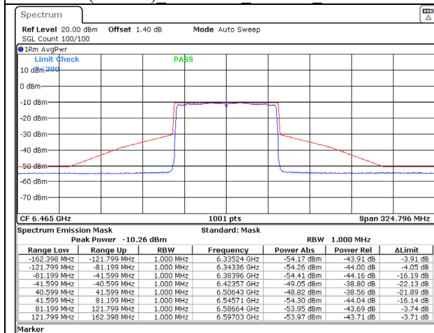
802.11ax (80MHz) 6465MHz Chain A NSS-1
