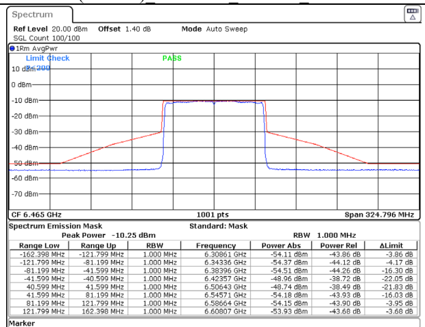
802.11ax (80MHz) 6465MHz Chain B NSS-1
