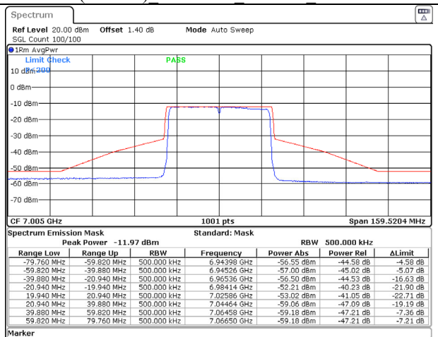
802.11ax (40MHz) 7005MHz Chain D NSS-1
