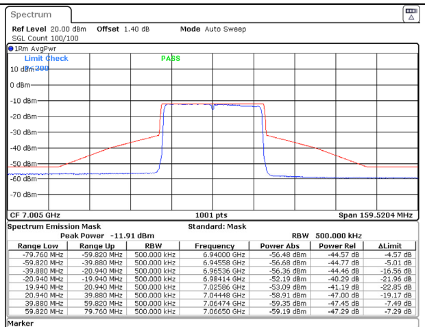
802.11ax (40MHz) 7005MHz Chain B NSS-1
