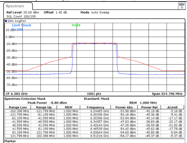
802.11ax (80MHz) 6385MHz Chain B NSS-1
