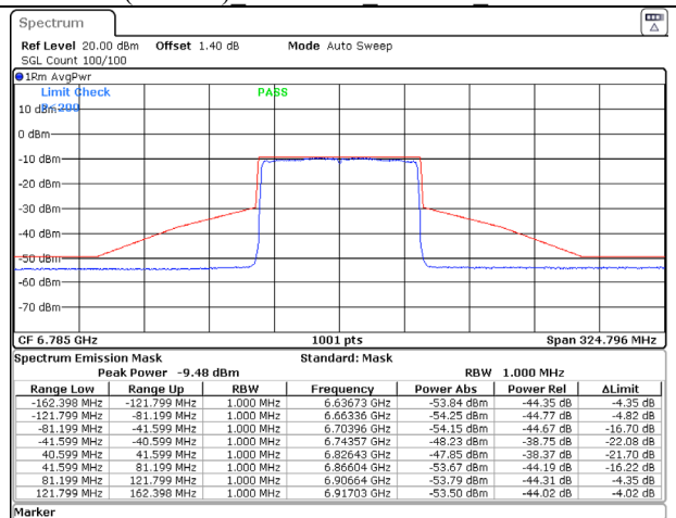
802.11ax (80MHz) 6785MHz Chain D NSS-1
