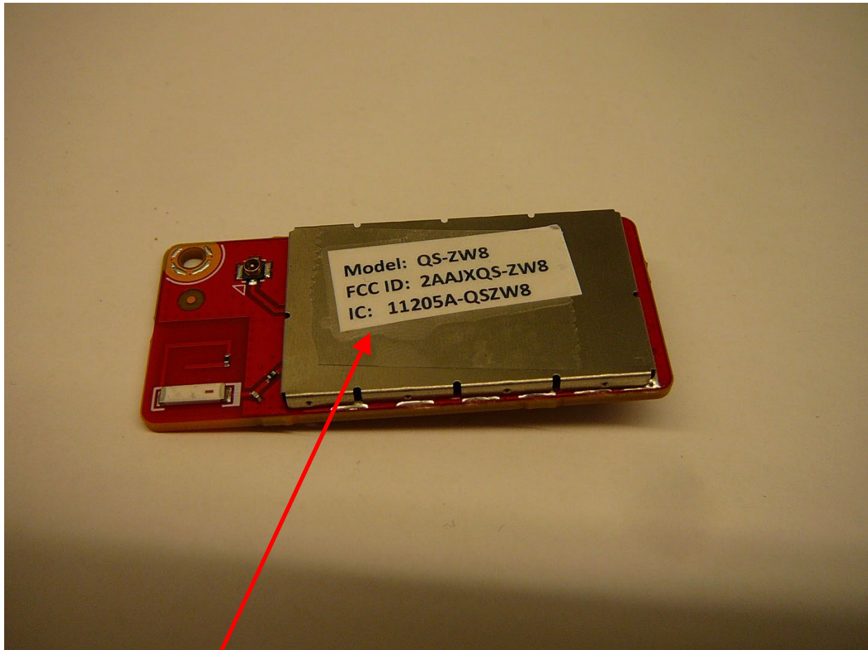
QS-ZW8 – Label
