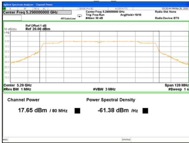
5290MHz_PK_Ant A
