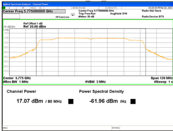
5775MHz_PK_Ant B
