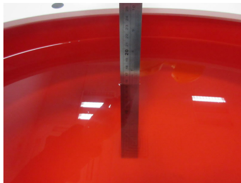
HSL1900MHz-2600MHz_16cm
