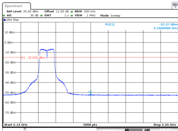
a_5200MHz_Chain 0
