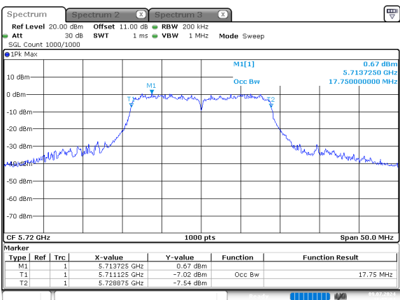
n20_5720MHz_Chain 0
