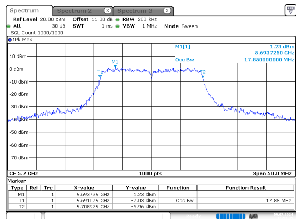
n20_5700MHz_Chain 0
