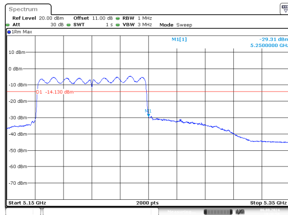
ac80_5210MHz_Chain 0
