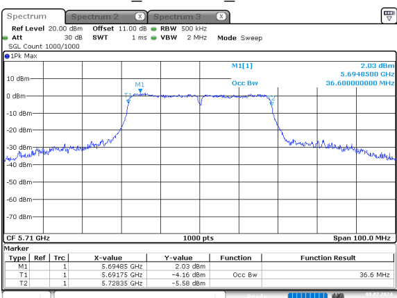
n40_5710MHz_Chain 0
