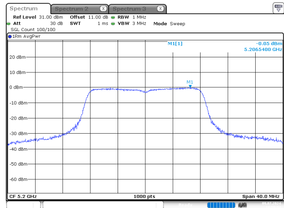
a_5200MHz_Chain 0
