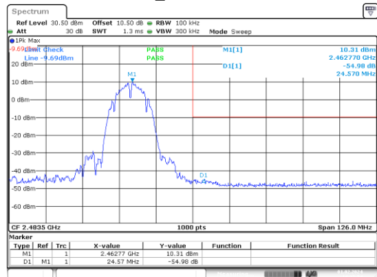
b_2462MHz
