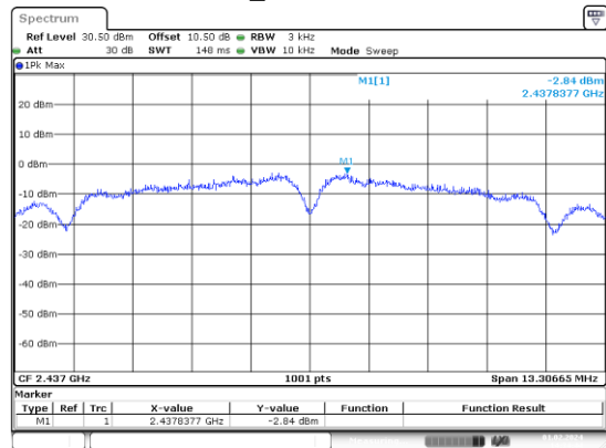
b_2437MHz
