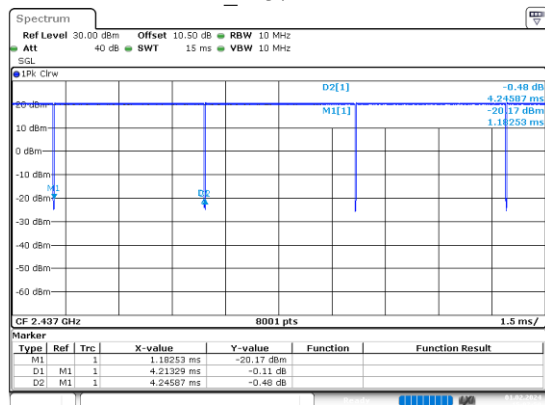
b_2437MHz
