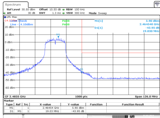
g_2462MHz
