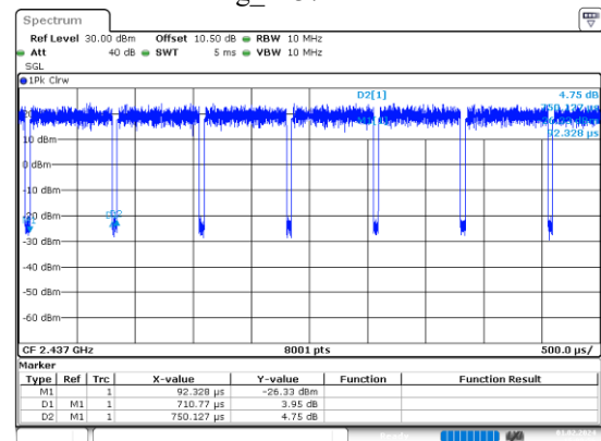
g_2437MHz
