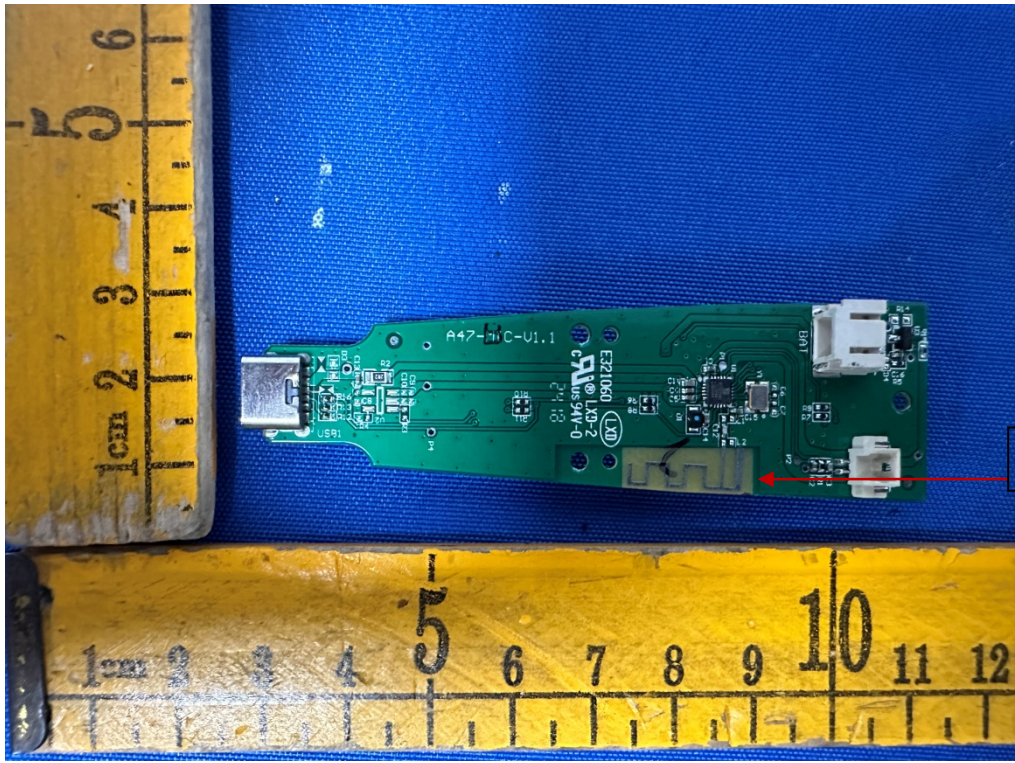
BLE Antenna
