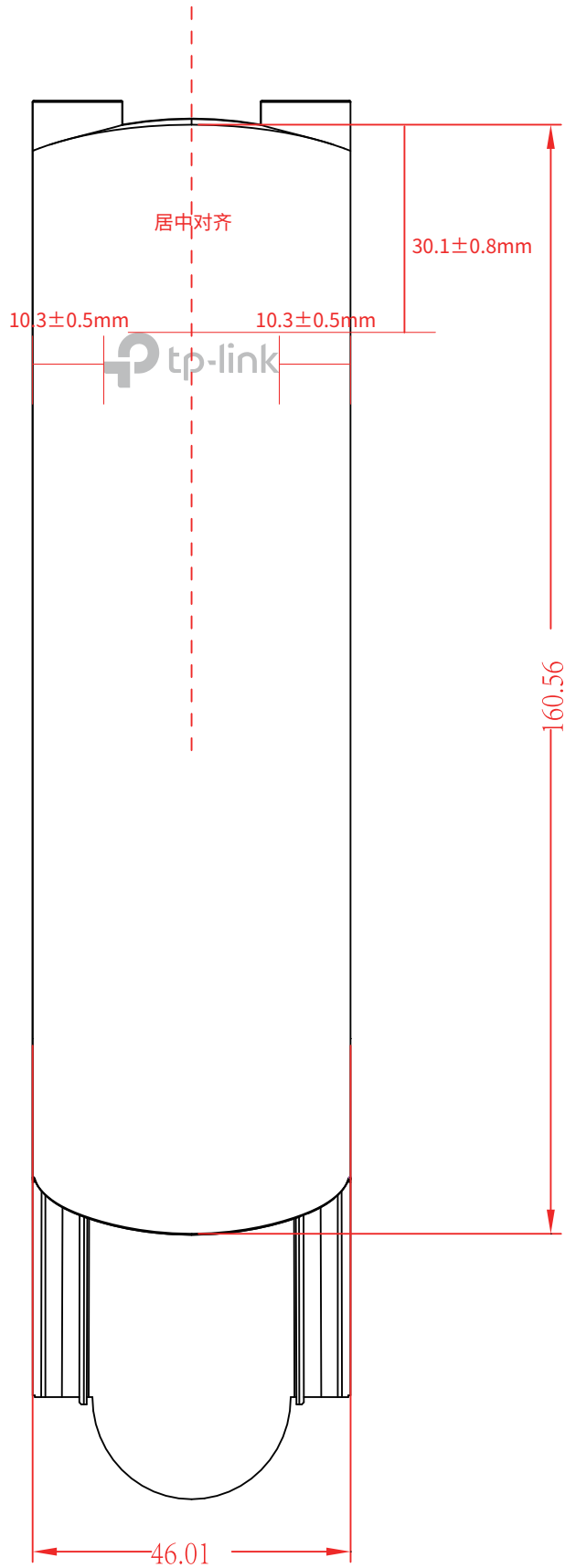
尺寸图
