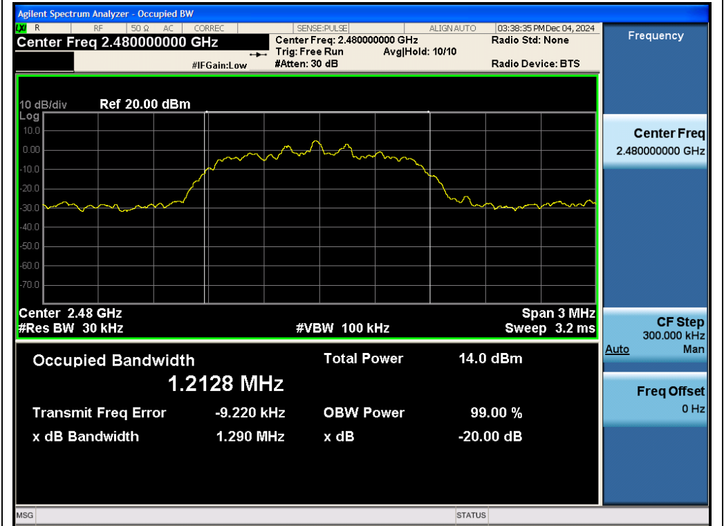
Test_Graph_EDR_ANT1_2480_2Mbps_OBW
