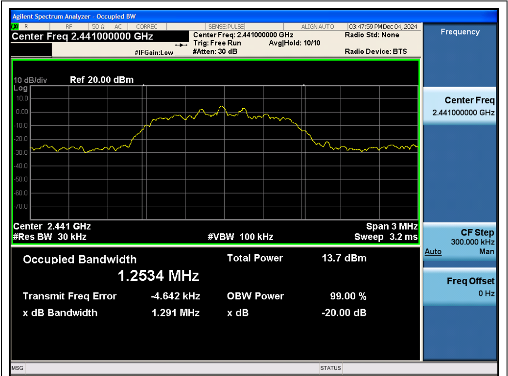
Test_Graph_EDR_ANT1_2441_2Mbps_OBW
