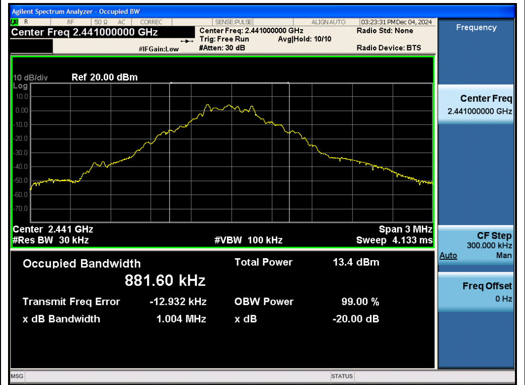
Test_Graph_BR_ANT1_2441_1Mbps_OBW
