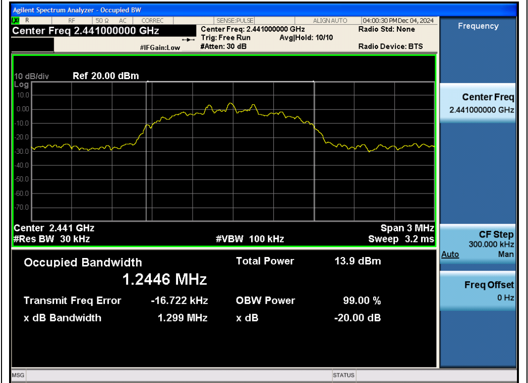
Test_Graph_EDR_ANT1_2441_3Mbps_OBW
