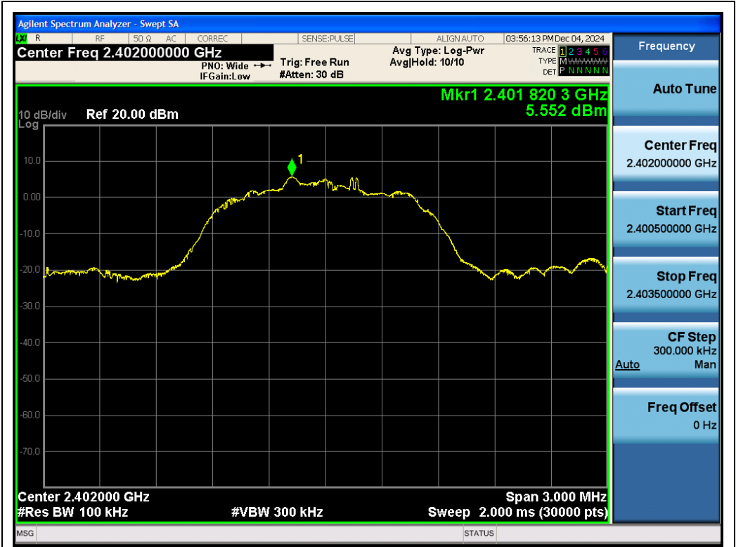
Test_Graph_EDR_ANT1_2402_3Mbps_Reference Level
