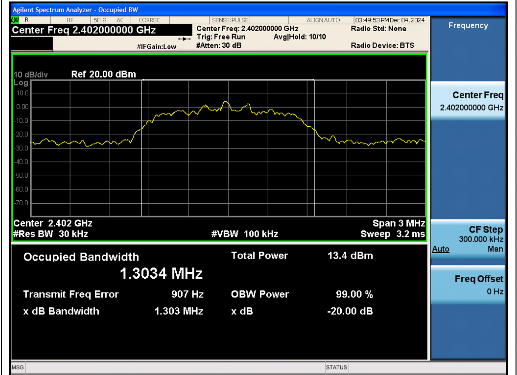
Test_Graph_EDR_ANT1_2402_2Mbps_OBW
