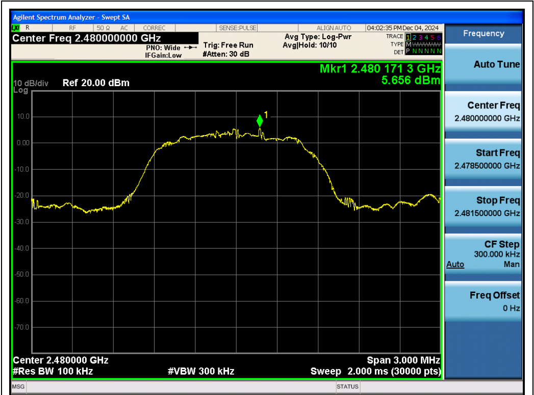
Test_Graph_EDR_ANT1_2480_3Mbps_Reference Level
