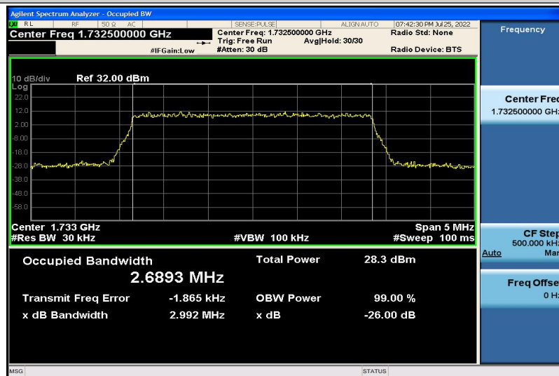
Band4-3MHz-QPSK-20175-15RB#0-2.6893
