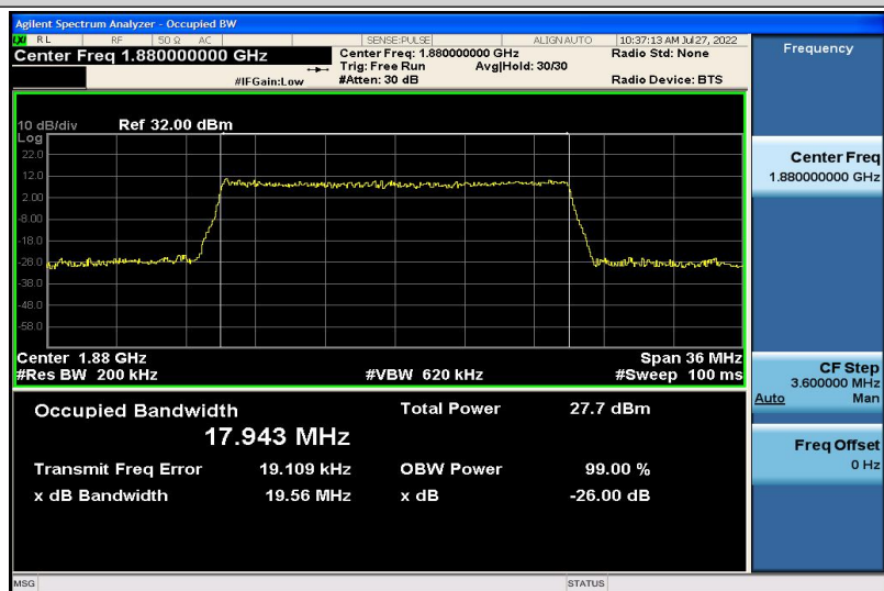
Band2-20MHz-QPSK-18900-100RB#0-17.943
