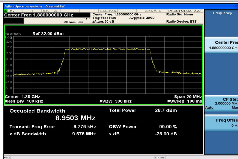
Band2-10MHz-QPSK-18900-50RB#0-8.9503
