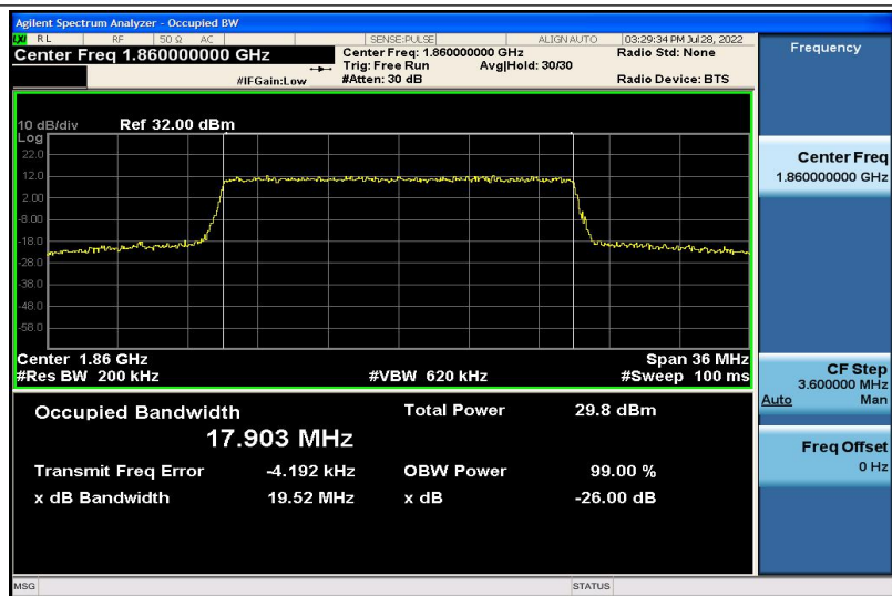
Band2-20MHz-QPSK-18700-100RB#0-9.1293
