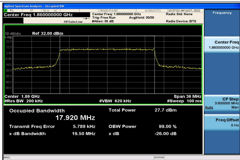
Band2-20MHz-16QAM-18700-100RB#0-17.920
