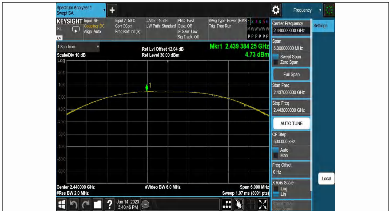
BLE_2M-Ant1-2440
