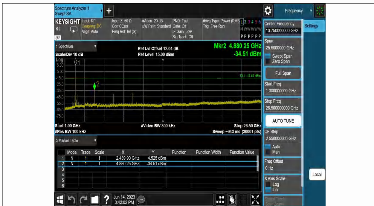
BLE 2M-Ant1-2440-1000~26500
