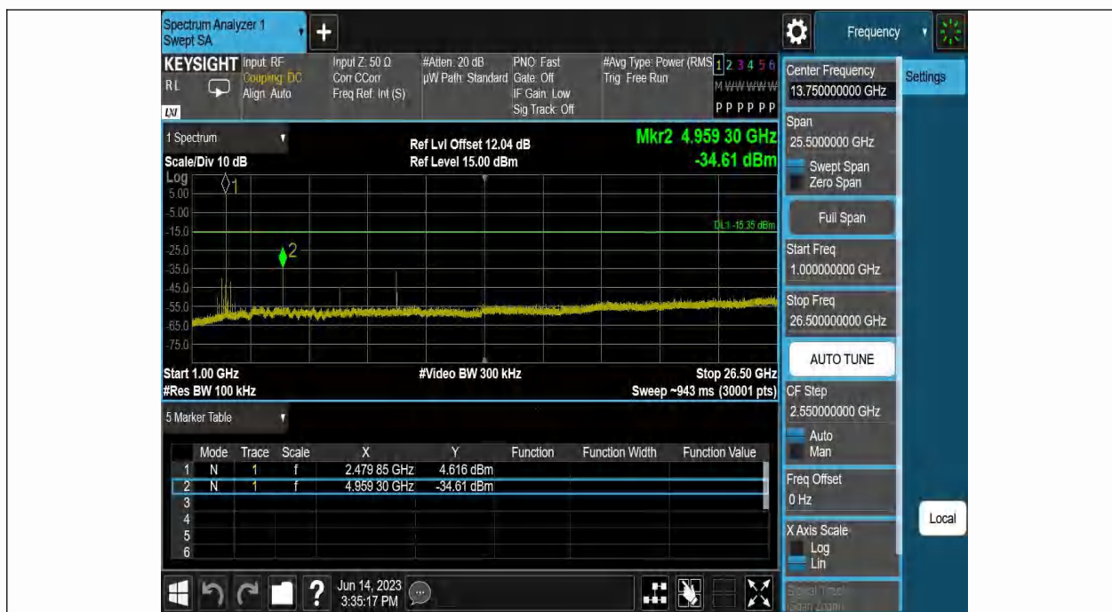
BLE 1M-Ant1-2480-1000~26500
