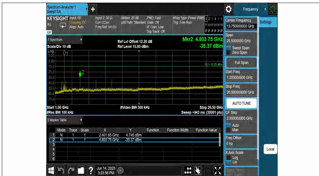
BLE 1M-Ant1-2402-1000~26500
