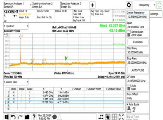
802.11ax_20MHz_Chain0_2437MHz_RU52_37
