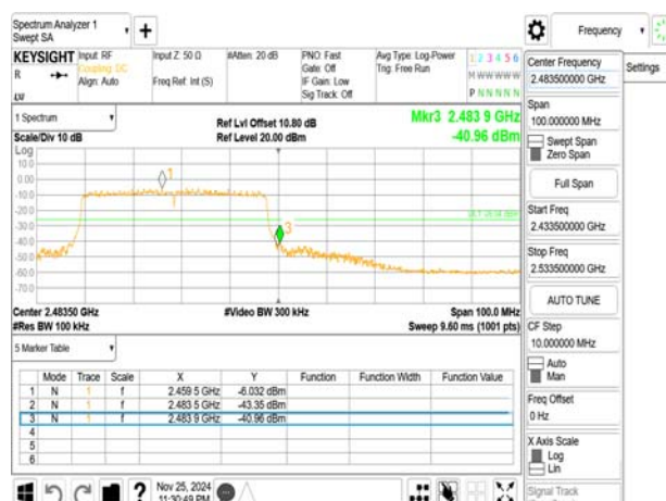
802.11ax_40MHz_Chain0_2462MHz_RU484
