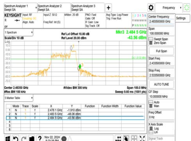
802.11ax_20MHz_Chain0_2472MHz_RU52_40
