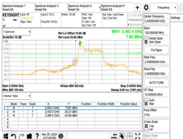
802.11ax_20MHz_Chain0_2412MHz_RU52_37
