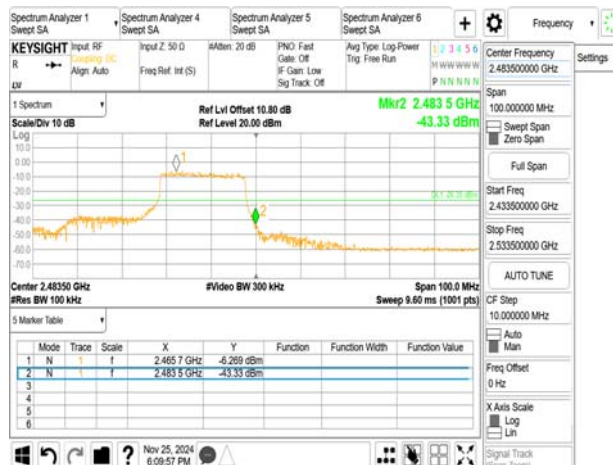
802.11ax_40MHz_Chain0_2462MHz_RU484
