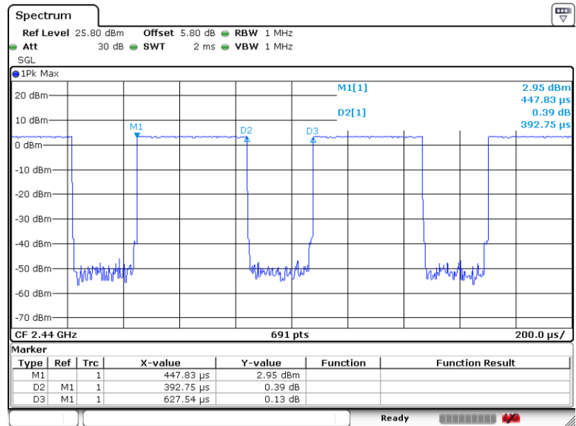
Bluetooth - LE1Mbps
