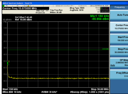
0.15MHz~30MHz
