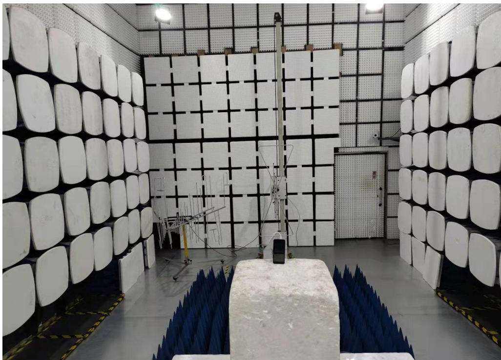
Fig. 1 (Below 1GHz)
