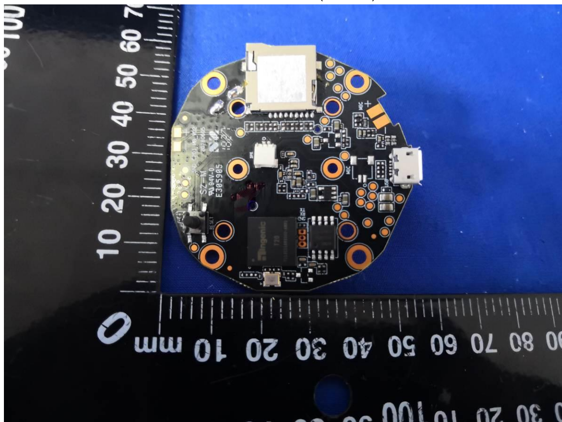
Mainboard-Rear View(SVC562)
