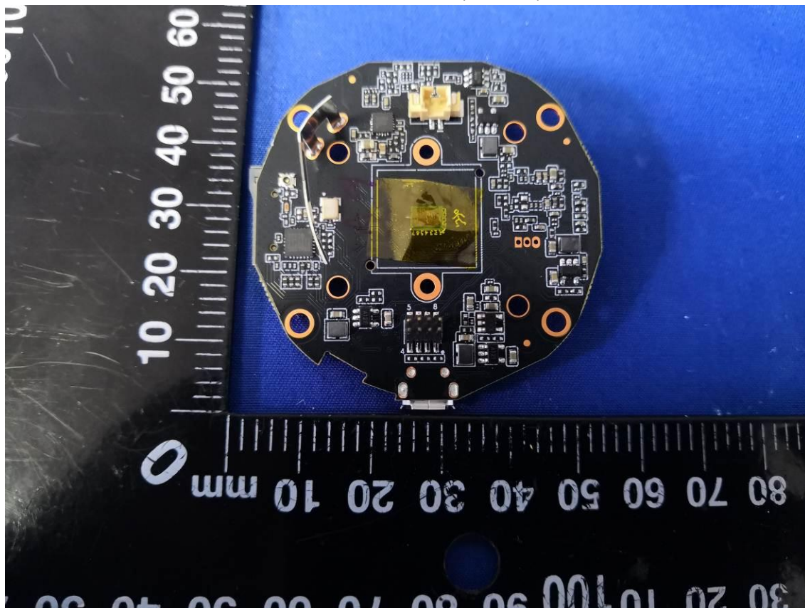
Mainboard-Front View(SVC562)
