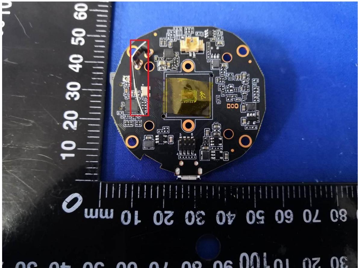
Antenna View(SVC562)
