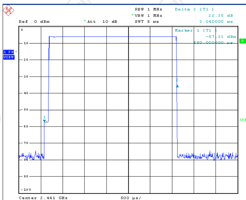
2441 MHz_DH5
