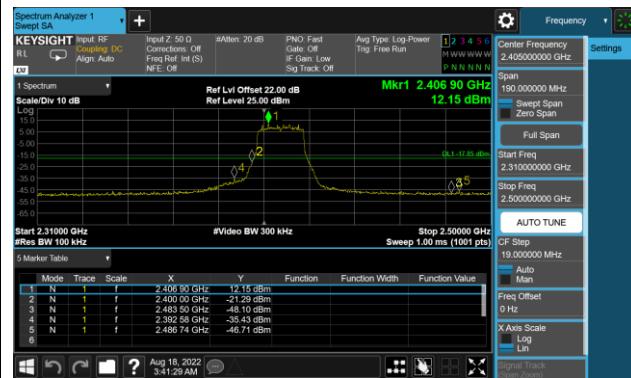
802.11 ax20 CH01 (2412MHz)
