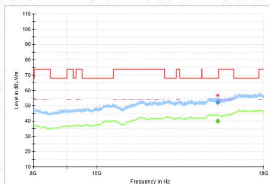
RSE-11AC-CH165-8GHz-18GHz
