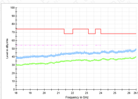
RSE-11AC(40M)-CH151-18GHz-26.5GHz
