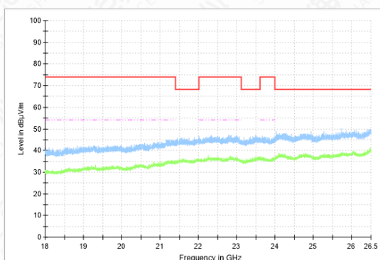
RSE-11AC-CH165-18GHz-26.5GHz
