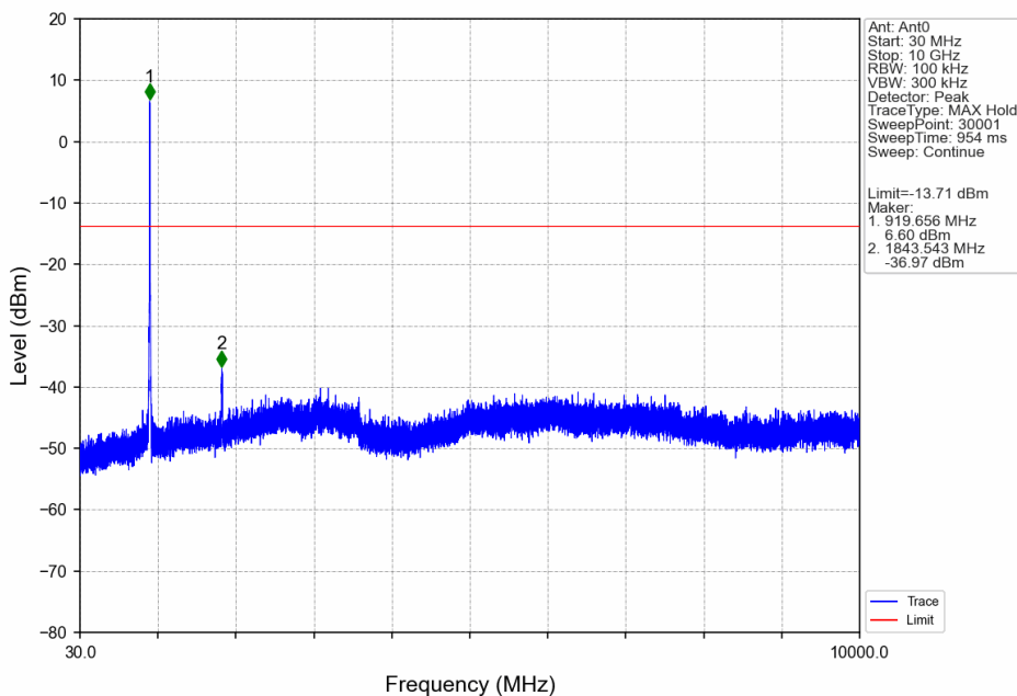
10M_HCH_923MHz_Ant0_NTNV
