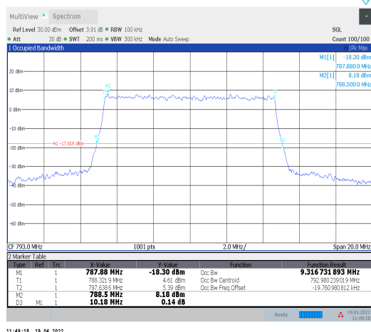
1-N14--15-10-M-9-CP-256QAM-Outer_Full-52@0-A nt0-9.317-10.180-≤10-PASS
